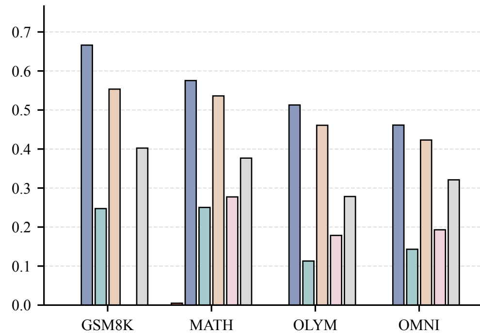
F1 Score
