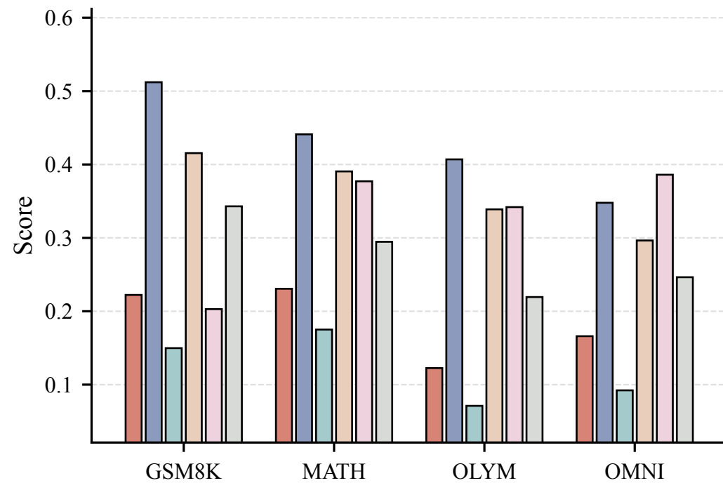
Error Acc
