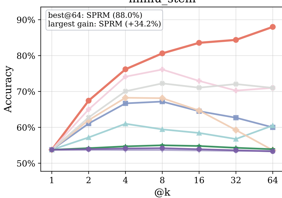
mmlu_stem
