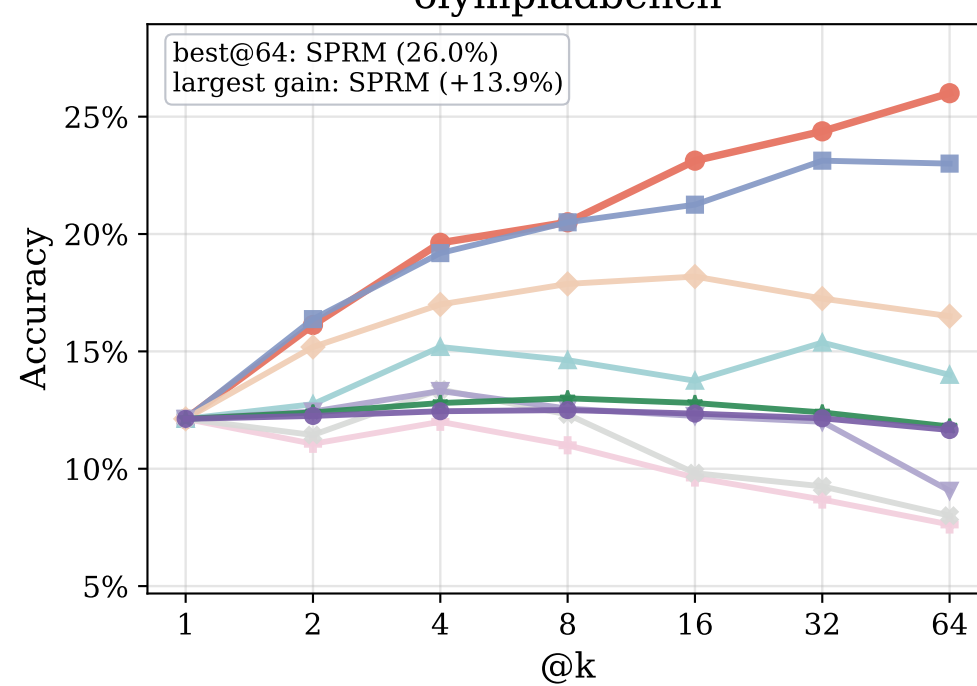
olympiadbench
