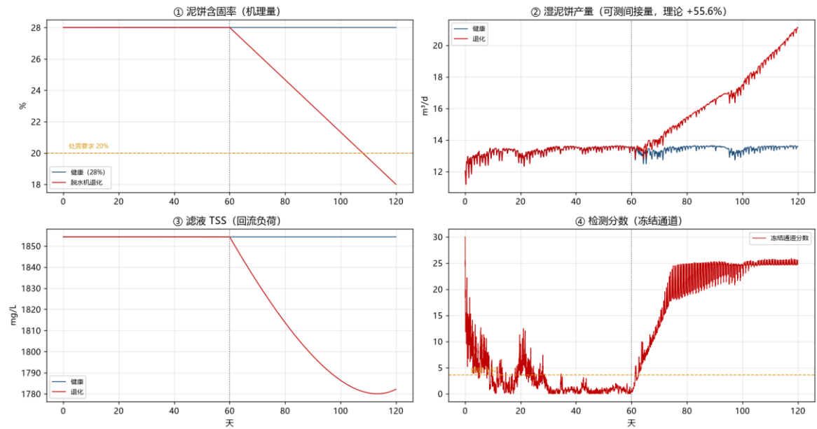
图 27 污泥线闭环（路线 A）：含固率、湿泥饼量、滤液与检测分数
