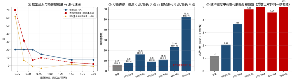
图 19 BSM1 退化幅值-斜率扫描：首报与幅值无关（严重度需另算）
