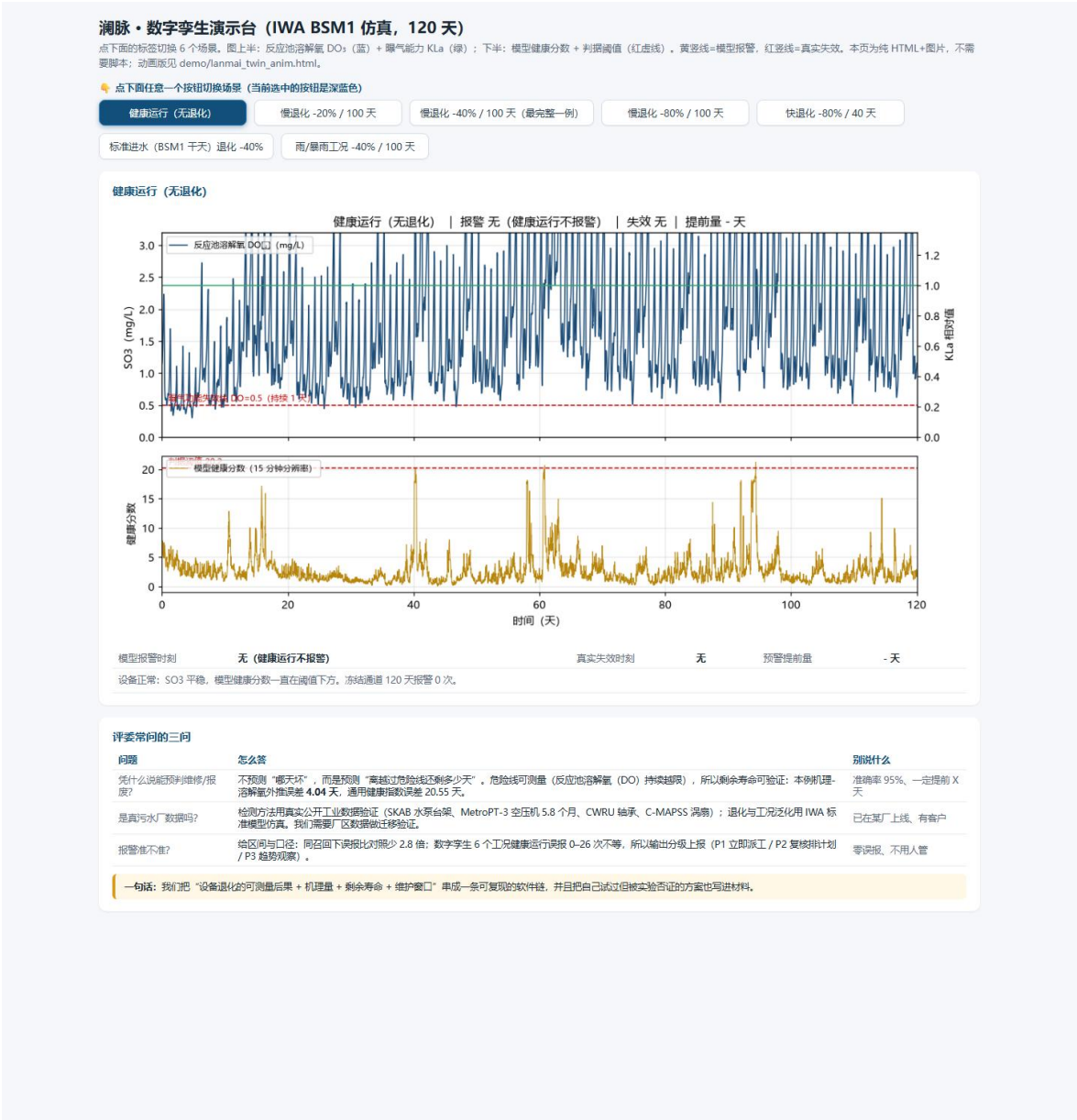
图 5 交互式数字孪生演示台（静态版）
