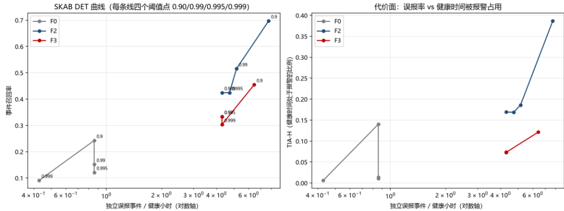
图 15 SKAB 检测误差权衡 (DET) 曲线: 三种方法
