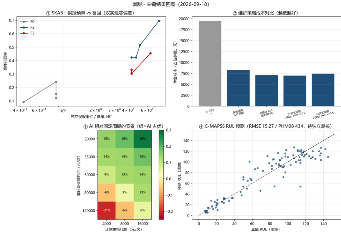
图 14 真实数据四图：误报-召回 / 策略成本 / 敏感性 / RUL 散点
