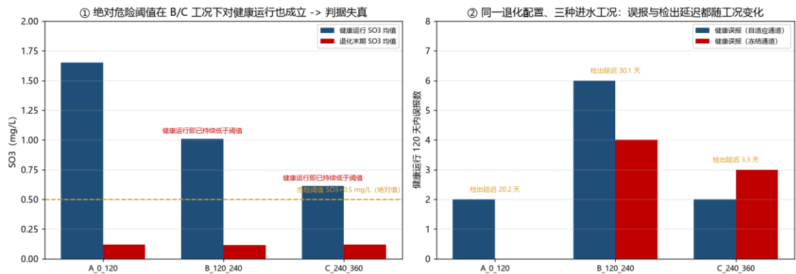
图 20 进水工况泛化：绝对阈值跨工况失效
