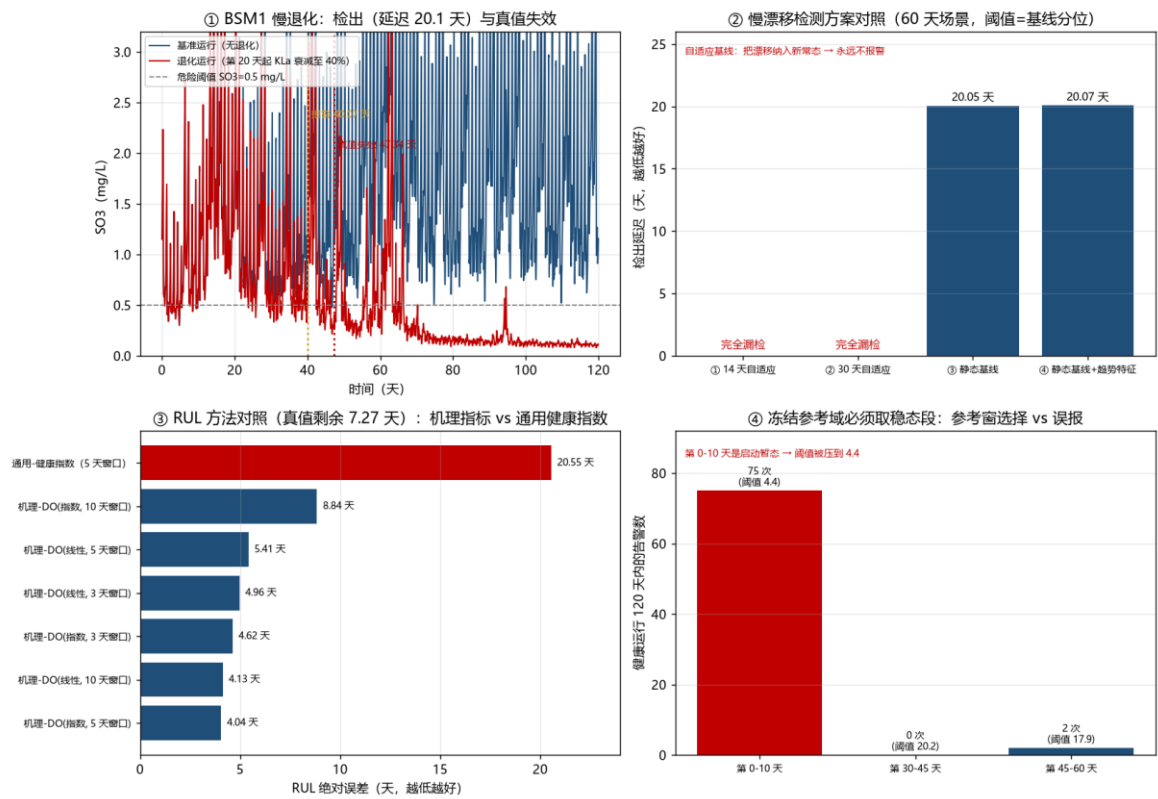
图 18 BSM1 数字孪生闭环四图：注入 → 检测 → RUL → 决策
