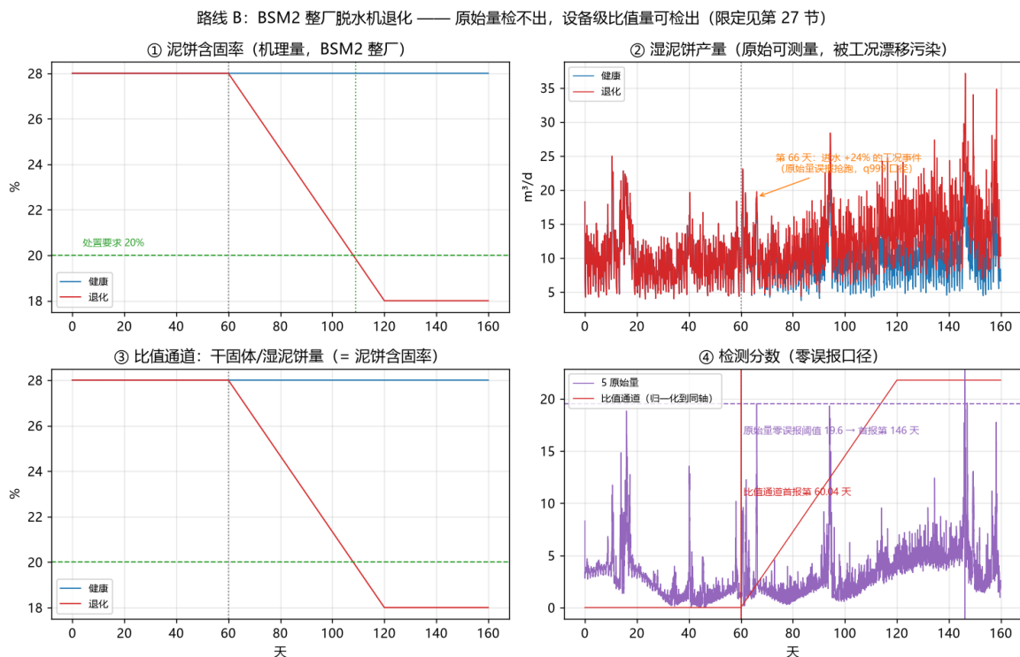
图 30 BSM2 整厂退化：原始量检不出、设备级比值通道可检出
