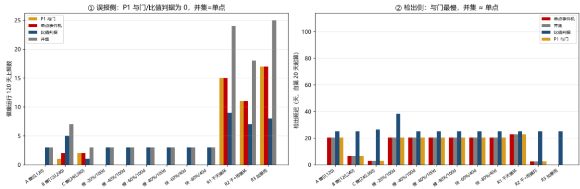
图 26 组合报警策略（单点/比值/并集/与门）对比
