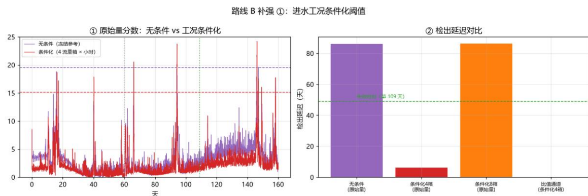
图 32 补强①: 工况条件化与同工况对拍差分的延迟对比
