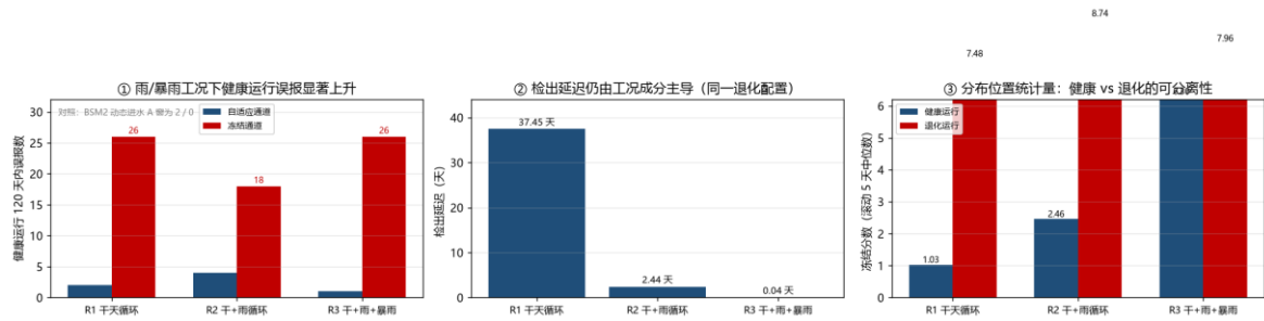
图 21 雨/暴雨冲击工况：工况事件必须单独处理
