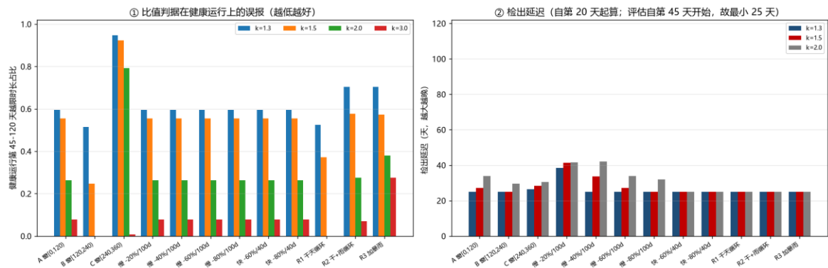
图 22 比值判据跨工况检验
