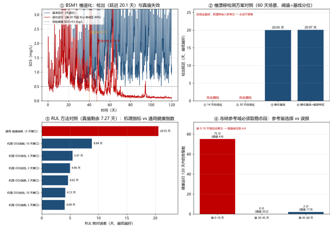
图 1-9 BSM1 数字孪生闭环四图：注入 → 检测 → RUL → 决策
