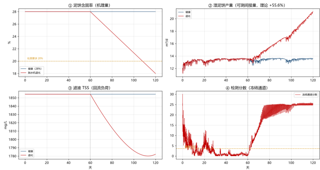
图 1-17 污泥线闭环（路线 A）：含固率、湿泥饼量、滤液与检测分数
