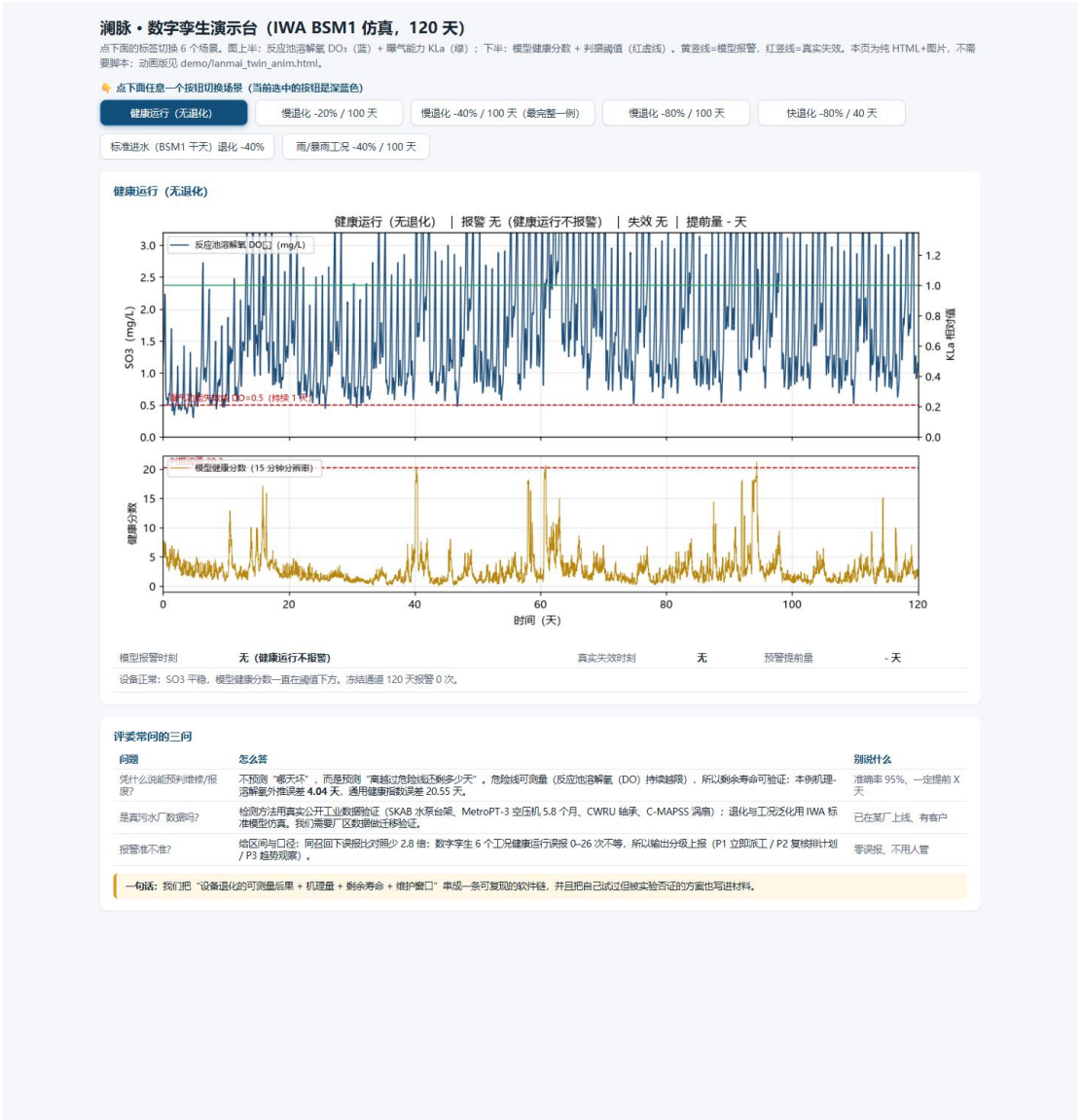
图 1-37 交互式数字孪生演示台（静态版）
