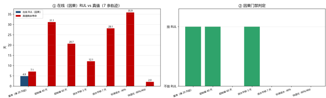
图 1-15 在线链路多轨迹：门禁挂载与在线 RUL 可算性
