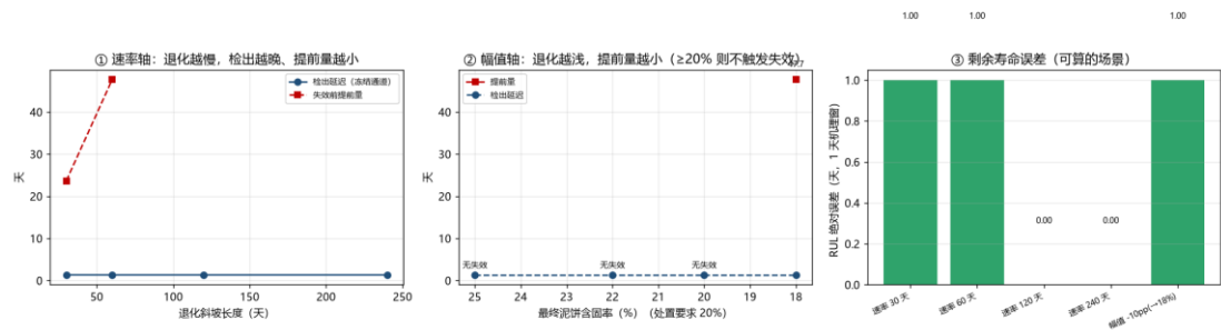
图 1-18 污泥线幅值/速率扫描：8 场景首报一致
