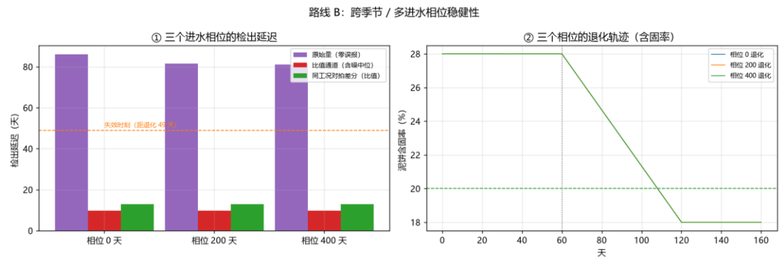
图 1-23 跨相位稳健性：三个进水相位结论一致
