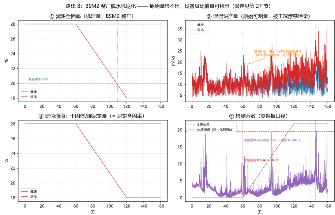
图 1-20 BSM2 整厂退化：原始量检不出、设备级比值通道可检出
