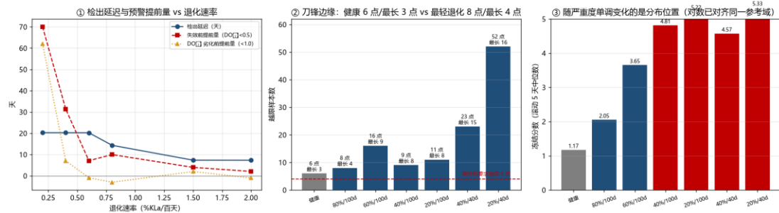
图 1-10 BSM1 退化幅值-斜率扫描：首报与幅值无关（严重度需另算）
