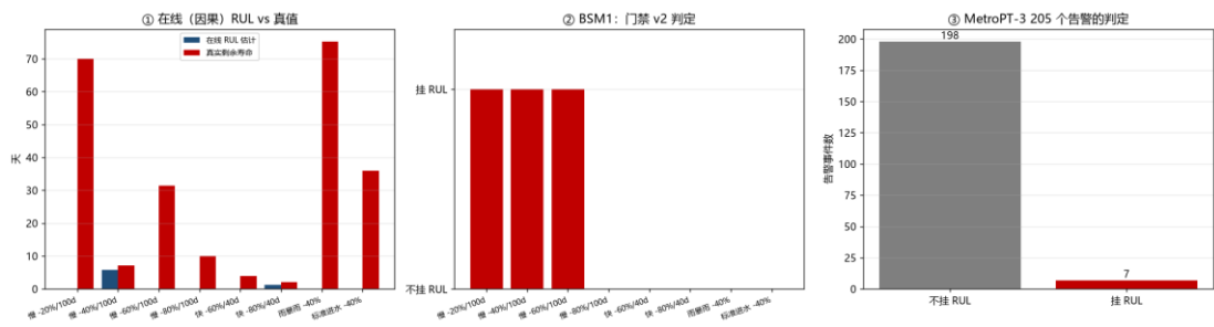
图 1-14 在线因果 RUL 门禁：判据与误挂率
