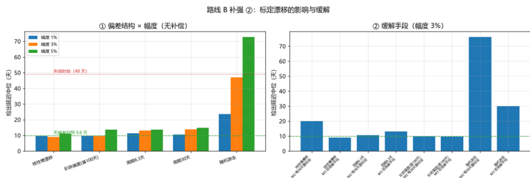
图 1-24 补强②：标定漂移的结构 × 幅度 × 缓解手段
