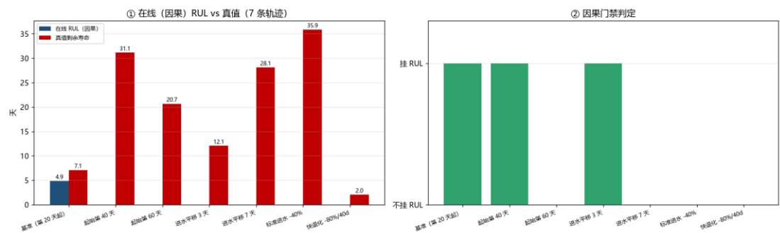
图 3-2 在线因果 RUL 门禁：判据与误挂率
