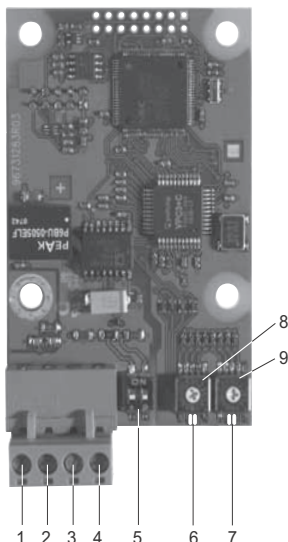
Fig. 1 CIM 1XX Profibus module
