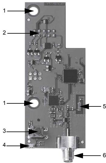
Fig. 1 CIM 060
