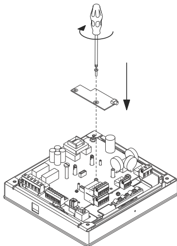
Fig. 4 Fitting the CIM 060 in the CU 362
