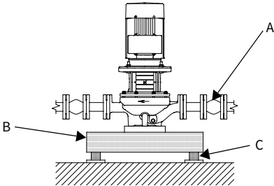
图 11 TP水泵基座
