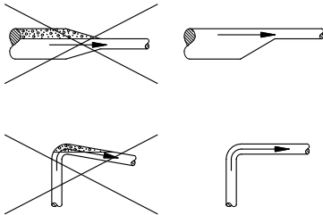
图 10 在水泵的吸水侧安装正确的管道。
