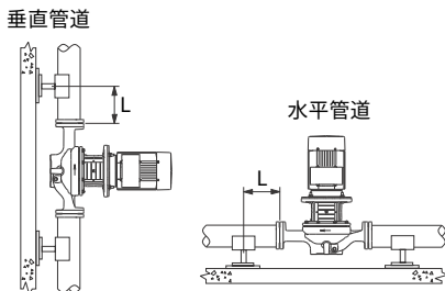
图6 直接悬挂在管道中的泵
