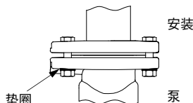
图5 在椭圆螺栓孔上使用垫圈
