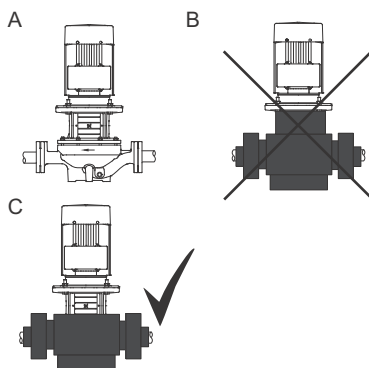
图 14 TP泵隔离
