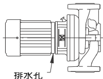
图 9 电机法兰的排水孔
