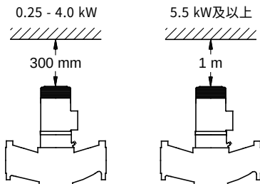
图 7 电机上方的空隙
