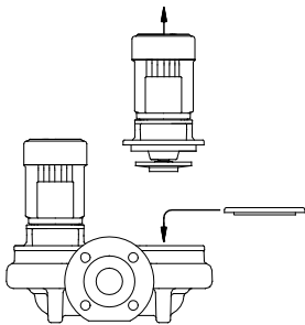
图 18 安装盲板法兰
