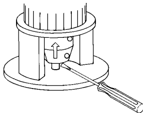
图 16 抬起联轴器和水泵轴
