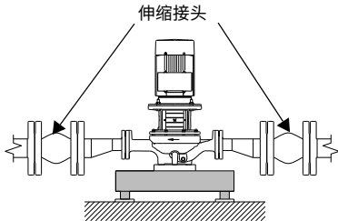
图 12 安装较大的伸缩接头的TP水泵
