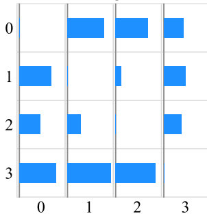
(d) bar in cell length
