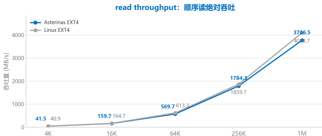
(a) 顺序读绝对吞吐: Asterinas与Linux EXT4对比
