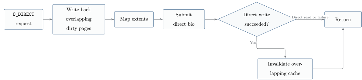
图 4-3 O_DIRECT请求与页缓存一致性处理路径
