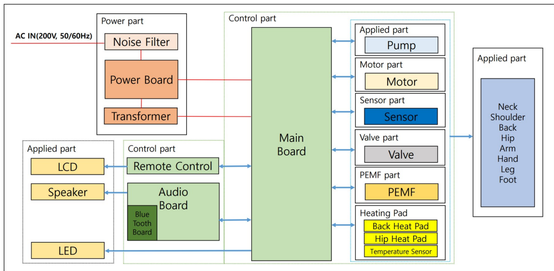
<그림 4> 안마의자의 작동원리(작동계통도)(출처 : 바디프랜드)
