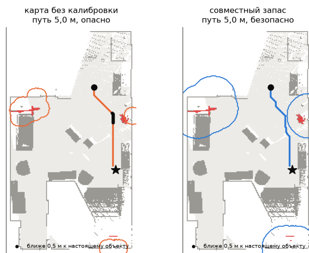
Рис. 2: Трудная задача при дрейфе L2 в системе координат планировщика. Красное — истинные растение и велосипед, линия — граница запретной зоны. Без калибровки зона не накрывает обрезанный край растения, и путь проходит ближе 0,5 м к нему (чёрные точки)
