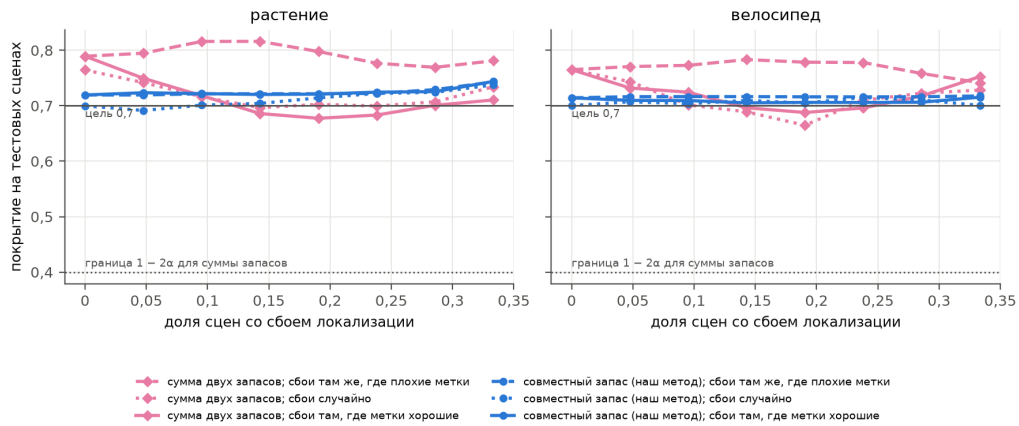
Рис. 3: Покрытие суммы отдельных запасов и совместного запаса в зависимости от доли сцен со сбоем локализации; 1 - \alpha = 0,7 , пунктир — граница 1 - 2\alpha для суммы
