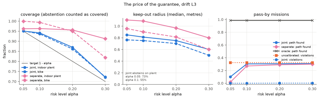
Рис. 6: Уровень риска \alpha против покрытия (слева, тонкая линия — номинал 1 - \alpha ), радиуса запаса (в центре) и исхода миссий (справа); дрейф L3, растение (сплошная) и велосипед (пунктир)
