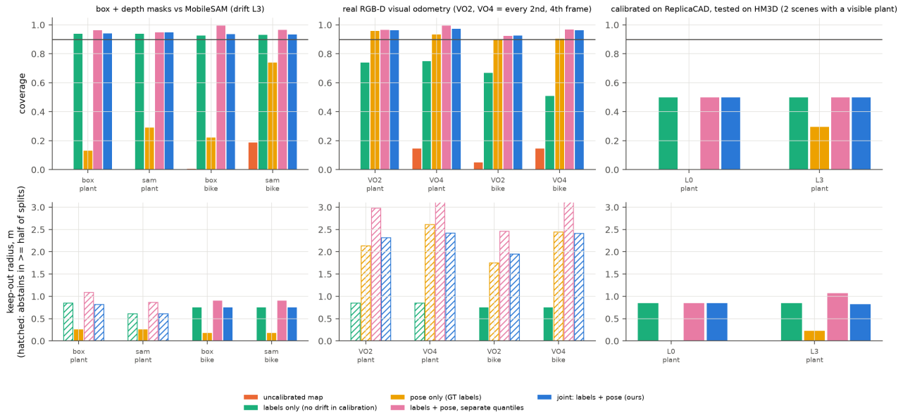
Рис. 8: Проверка упрощений: покрытие (сверху; линия — номинал 0,9) и медианный радиус (снизу; штриховка — ветка отказывается в половине разбиений или чаще) для масок MobileSAM, реальной визуальной одометрии и сцен HM3D
