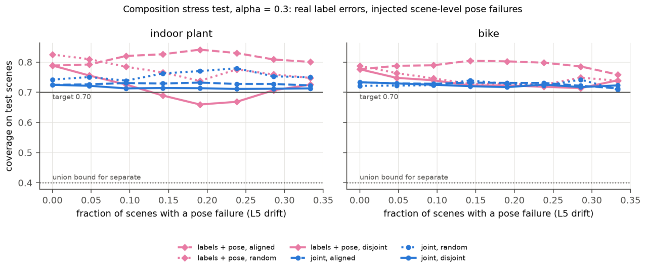
Рис. 7: Покрытие раздельной (розовая) и совместной (синяя) калибровки в зависимости от доли сцен с отказом локализации и от того, в каких сценах происходят отказы; \alpha = 0,3 , нижняя пунктирная линия — граница 1 - 2\alpha , которую гарантирует сумма квантилей
