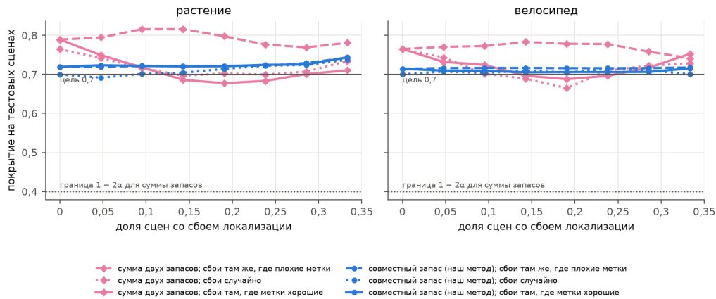
Рис. 4: Покрытие суммы отдельных запасов и совместного запаса в зависимости от доли сцен со сбоем локализации; 1 - \alpha = 0,7 , пунктир — граница 1 - 2\alpha для суммы
