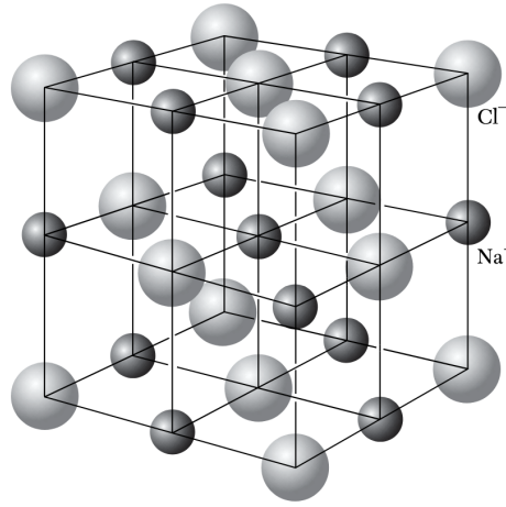
Abbildung 2.2: Schematische Darstellung des räumlichen Aufbaus des NaCl-Kristalls in drei Dimensionen. Abbildung entnommen aus [10, S. 13].
