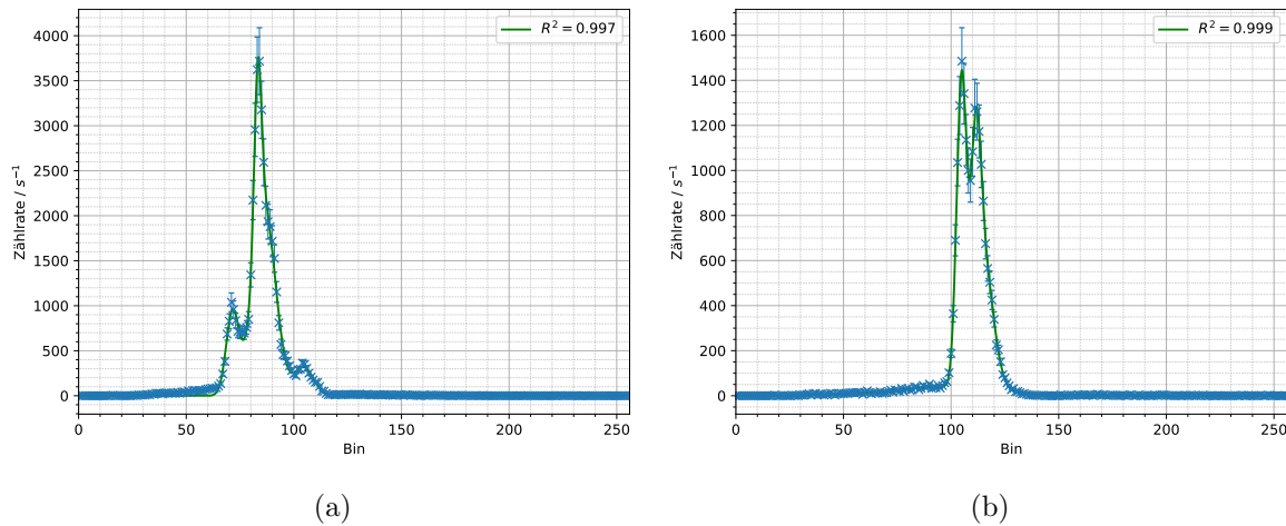
Abbildung 3.4: a) Messung und Anpassung von Gausskurven für Probe 1 und b) Probe 2
