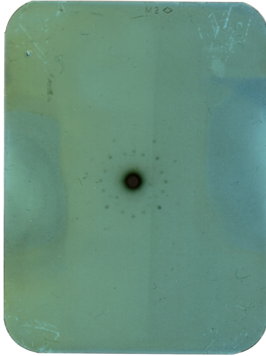
Abbildung 4.1: Scan der Laue Aufnahme
