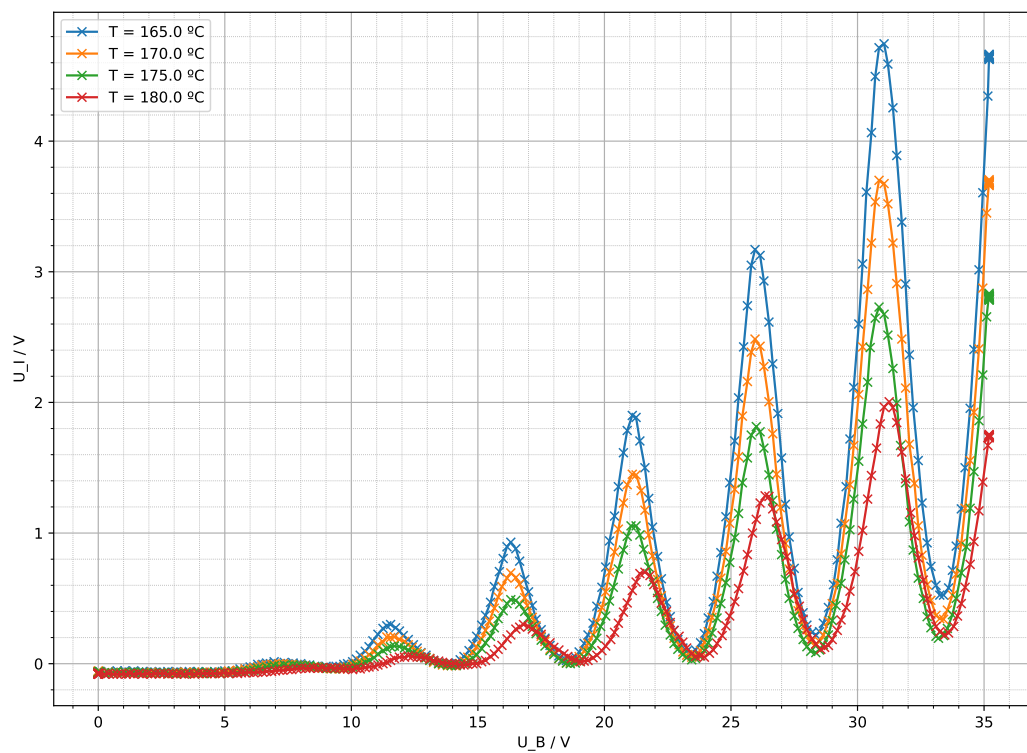
Abbildung 1.3: Messungen bei verschiedenen Temperaturen und U_G = 2,5 V.
