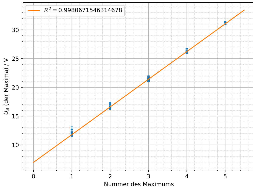
Abbildung 3.4: Auftragung der Daten aus ?? mit Anpassung einer Geraden. Die Unsicherheiten ergeben sich aus den Standardabweichungen der Anpassungsergebnisse.
