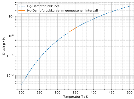
Abbildung 3.6: Dampfdruckkurve von Quecksilber nach dem funktionalen Zusammenhang von Temperatur und Druck in [12, S. 12]
