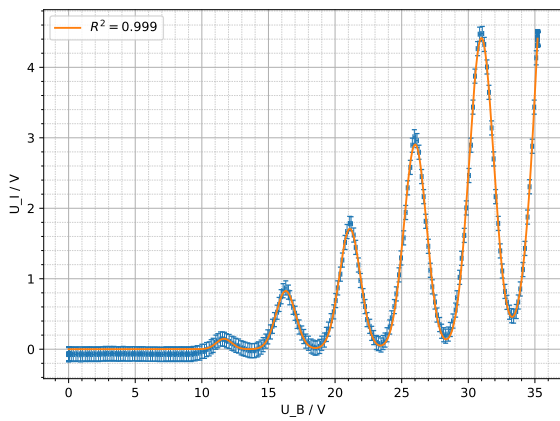
Abbildung 3.3: Beispielhafte Messkurve bei T = (165 \pm 2)^\circ\text{C} und U_G = (2,5 \pm 0,1) \text{ V} mit eingezeichneten Gaussfunktionen aus der Anpassung.
