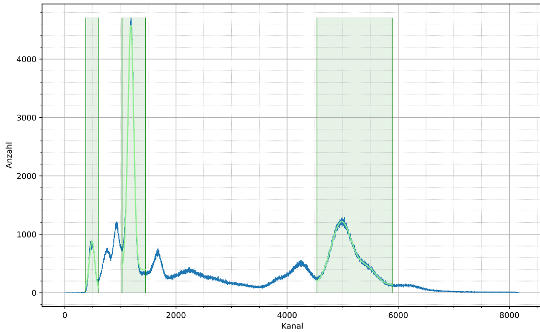
Abbildung 4.6: ^{133}\text{Ba} Spektrum, aufgenommen mit der linken Seite mit CFD als Gate. Die Parameter der eingezeichneten Anpassungen sind in [reference] gelistet. Die angepassten Linien sind nur zu illustrationszwecken vldr. die K_\alpha , 81,0 keV, 356,0 keV und die 383,8 keV Line. Dies kann anhand durch Vergleich mit Tabelle 3.3 gesehen werden.
