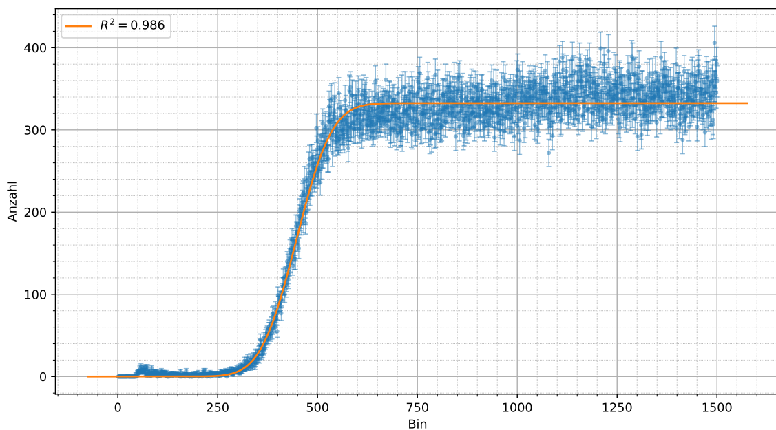
Abbildung 4.7: Anpassung zur Bestimmung der rechten CFD Schwelle, an die ersten 1500 Kanäle.
