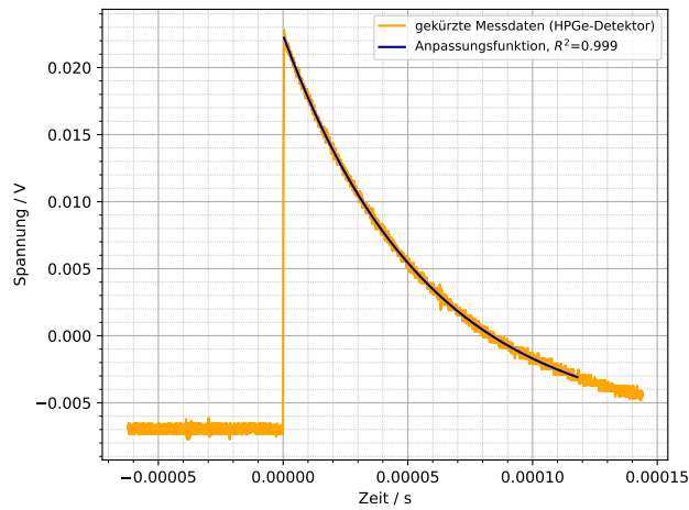
Abbildung 4.2: Ausschnitt der Aufnahme eines Oszilloskopsignals des HPGe-Detektors für ^{137}\text{Cs} mit angepasster Exponentialfunktion mit Parametern A = (0,0 \pm 1,6) \cdot 10^3 \text{ V} , b = (-17\,327 \pm 25) \text{ s}^{-1} , c = (-0,006\,880 \pm 0,000\,018) \text{ V} , t_0 = (0,00 \pm 0,87) \text{ s} sowie Bestimmtheitsmaß R^2 = 0,999 .
