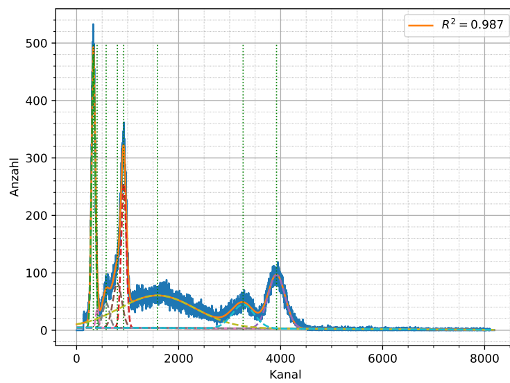
Abbildung 2.1: Bereitgestellte Daten mit Anpassungsfunktion mit eingezeichneten Amplitudenspitzen \mu_i und jeweiligen.
