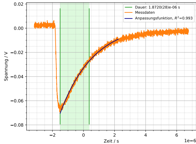
Abbildung 7.1: Oszilloskopaufnahme eines weiteren Anodendraht-Signals (in orange). Anpassungsparameter an die Anpassungsfunktion (in blau): a = (-4,668 \pm 0,061) \cdot 10^5 \text{ s}^{-1} , b = (3,85 \pm 0,45) \text{ mV} , c = (0,0 \pm 3,6) \cdot 10^4 \text{ V} , t_0 = (0,00 \pm 0,32) \text{ s} , als Dauer (grün hinterlegt) d = (1,8720 \pm 0,0028) \mu\text{s} .
