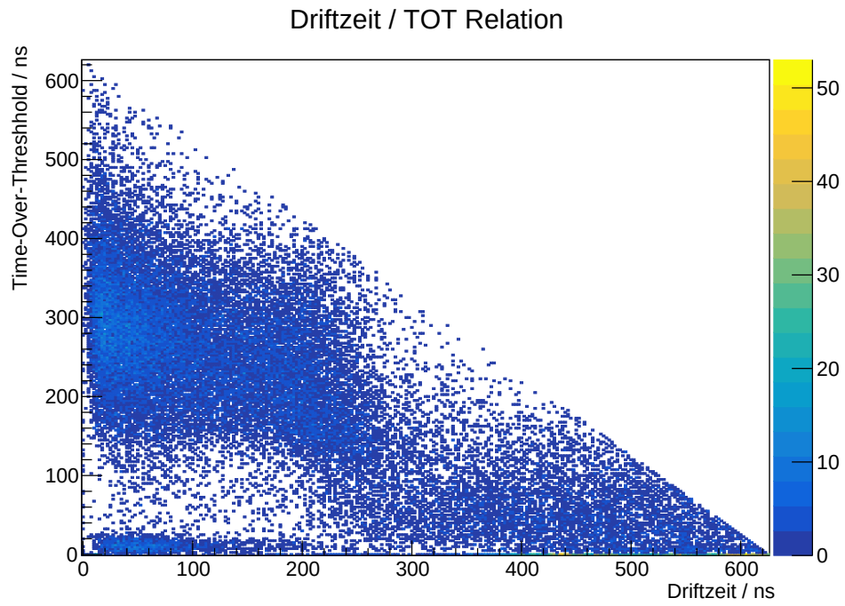
Abbildung 6.2: Driftzeit gegen TOT, ungefiltert
