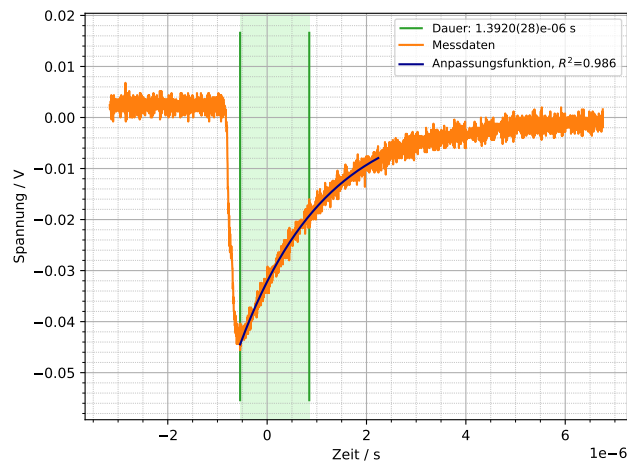
Abbildung 7.2: Oszilloskopaufnahme eines weiteren Anodendraht-Signals (in orange). Anpassungsparameter an die Anpassungsfunktion (in blau): a = (-5,76 \pm 0,13) \cdot 10^5 \text{ s}^{-1} , b = (1,26 \pm 0,52) \text{ mV} , c = (0,0 \pm 4,8) \cdot 10^4 \text{ V} , t_0 = (0,00 \pm 0,40) \text{ s} , als Dauer (grün hinterlegt) d = (1,3920 \pm 0,0028) \mu\text{s} .
