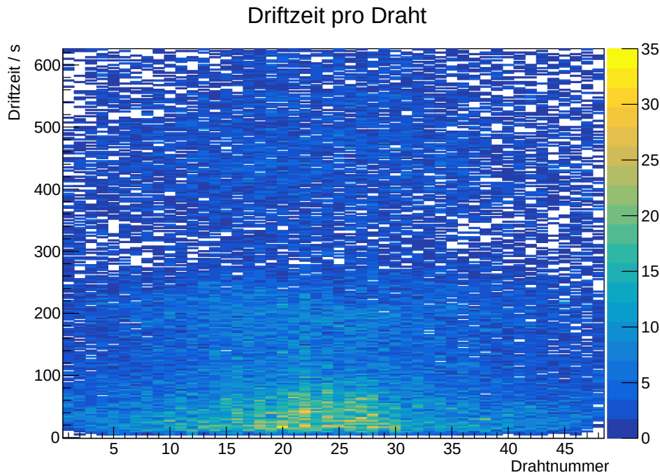
Abbildung 6.1: Driftzeiten pro Draht, ungefiltert
