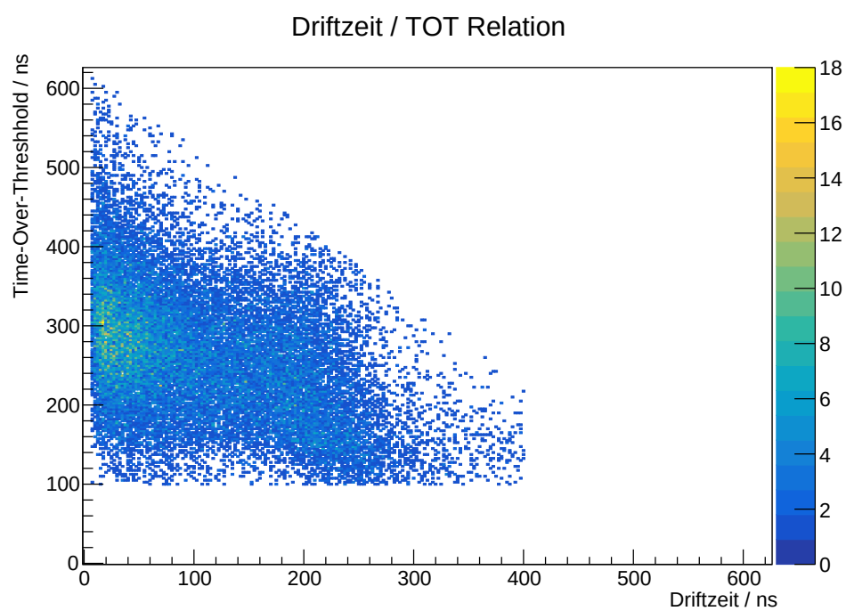
Abbildung 6.4: Driftzeit gegen TOT, gefiltert
