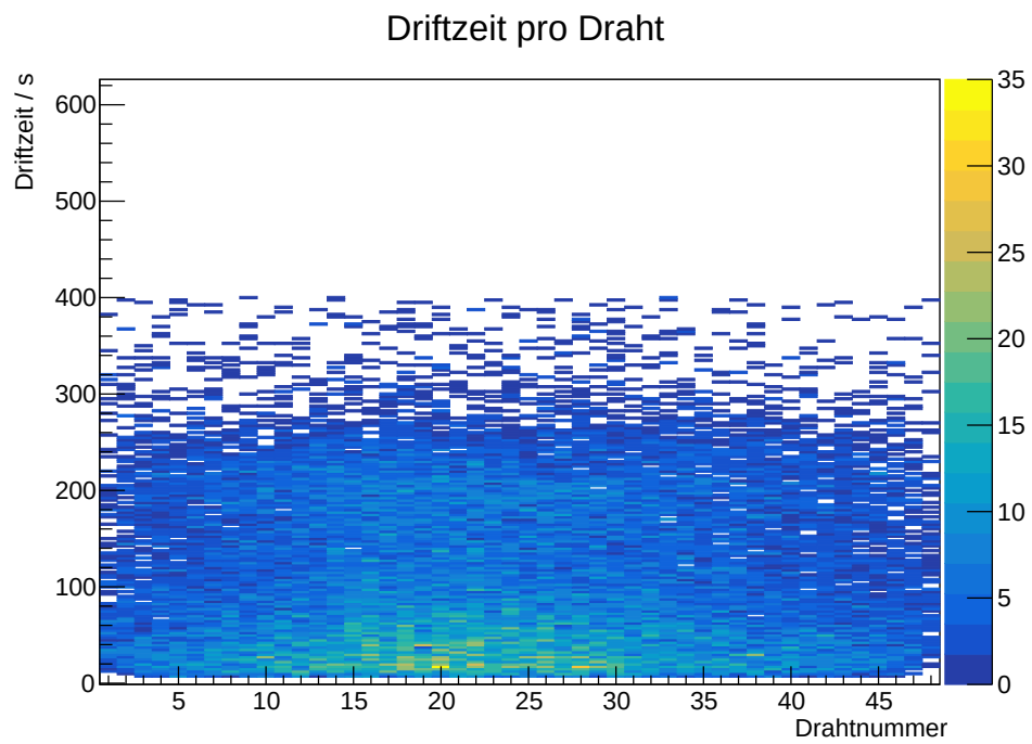
Abbildung 6.3: Driftzeiten pro Draht, gefiltert
