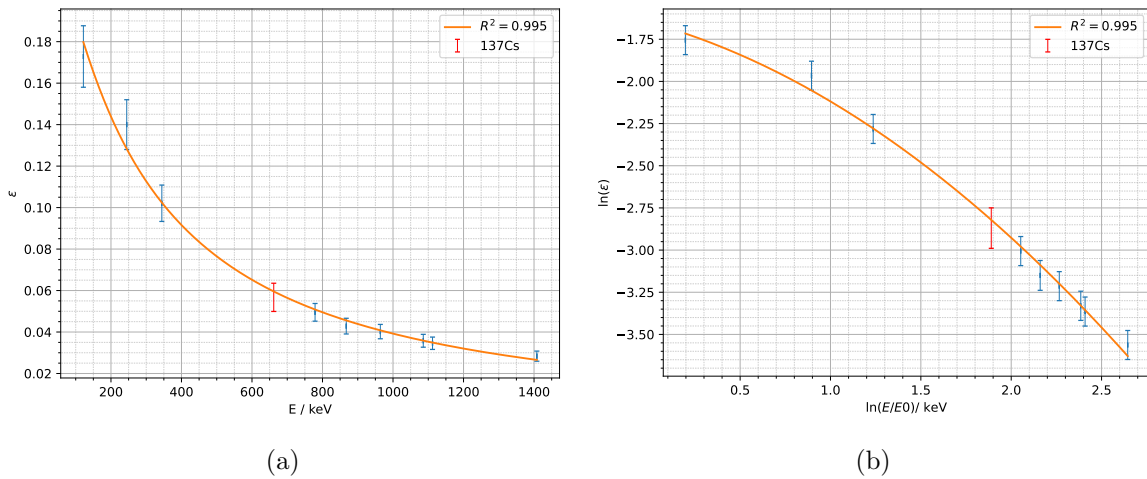
Abbildung 6.1: a) Effizienzkurve des HPGE Detektors mit Effizienz für Cäsium und Anpassungsfunktion eingezeichnet und b) Auftragung der Daten nach (6.8) an denen die Anpassung durchgeführt wurde.
