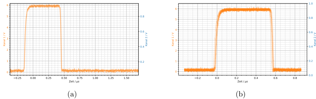
Abbildung 3.18: a) Lage des rechten SCA Signals relativ zum linken Trigger, welcher an der steigenden Flanke des rechten SCA lag, vor Anpassung der Verzögerung und b) nach Anpassung der Verzögerung
