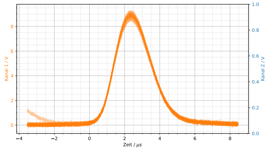
Abbildung 3.15: Linksseitige DA Signale, getriggert am linken SCA Ausgang, welcher nicht sichtbar ist.
