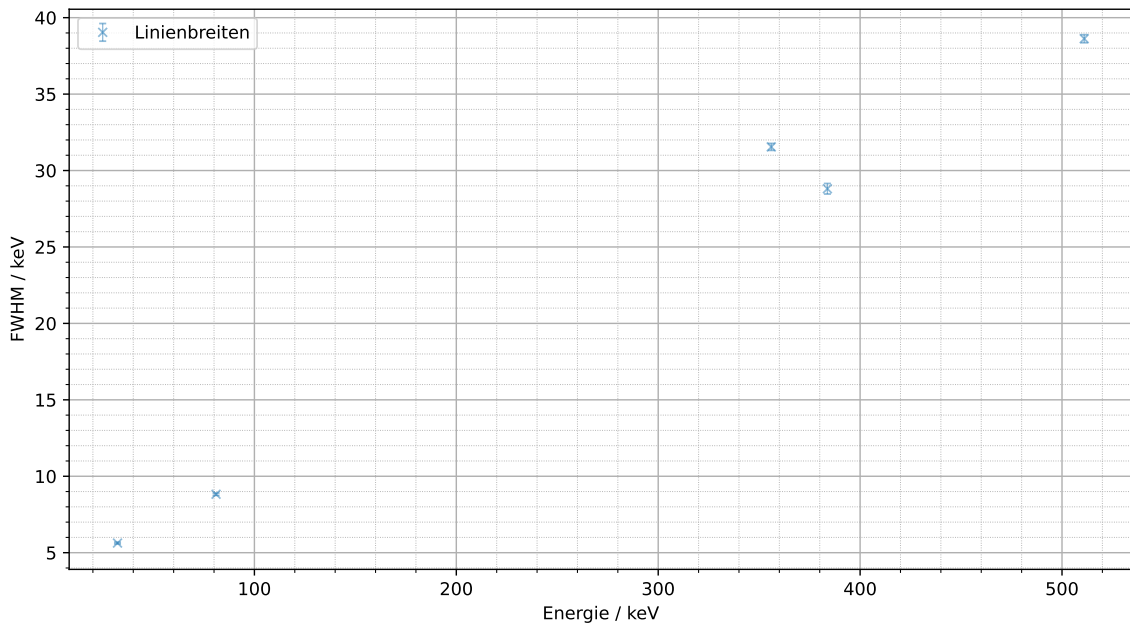
Abbildung 3.9: Linienbreiten gegen Energie der Linien des Linken Szintillators.
