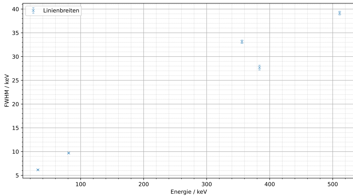
Abbildung 3.10: Linienbreiten gegen Energie der Linien des rechten Szintillators.
