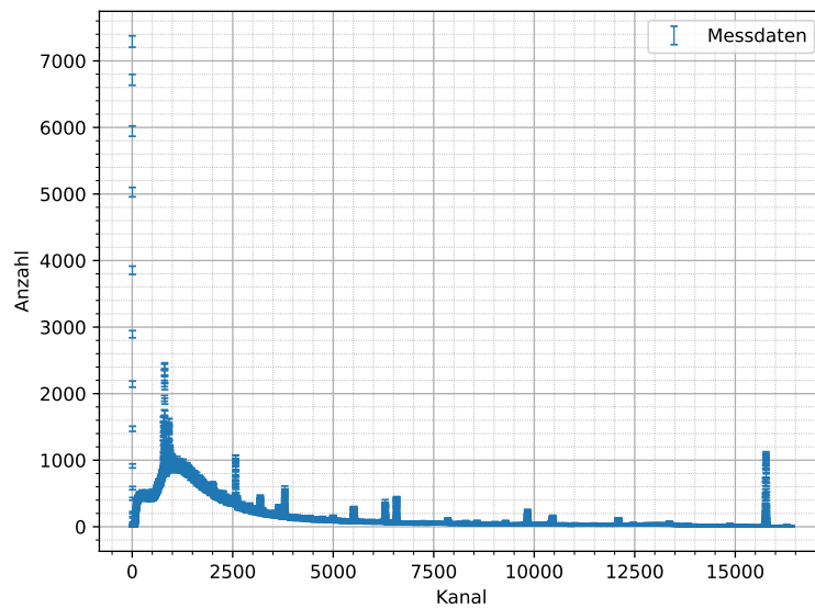
Abbildung 6.12: Mit HPGE-Detektor aufgenommenes Untergrundspektrum für die Bodenprobe, mit Fehler der Messanzahl N von \Delta N = \sqrt{N} , Messdauer: t = 18 h.
