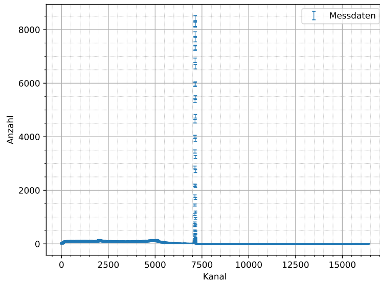
Abbildung 6.9: Mit HPGe-Detektor aufgenommenes Spektrum von ^{137}\text{Cs} mit Fehler der Messanzahl N von \Delta N = \sqrt{N} , Messdauer: t = 300 s.
