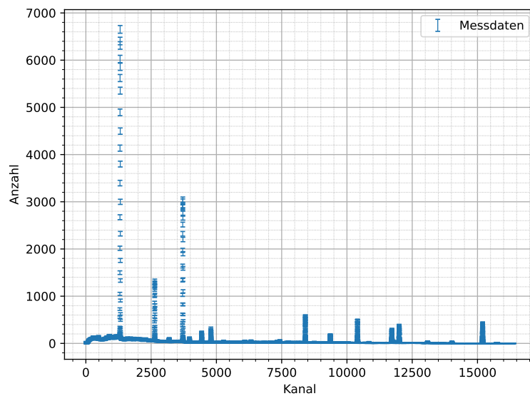
Abbildung 6.10: Mit HPGe-Detektor aufgenommenes Spektrum von ^{152}\text{Eu} mit Fehler der Messanzahl N von \Delta N = \sqrt{N} , Messdauer: t = 300 s.
