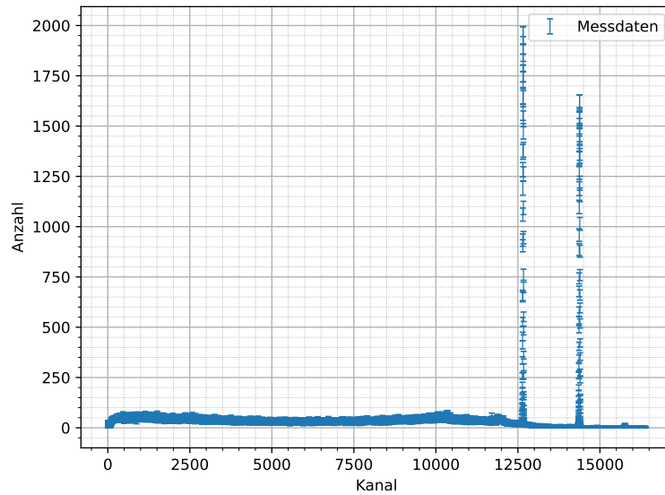
Abbildung 6.8: Mit HPGe-Detektor aufgenommenes Spektrum von ^{60}\text{Co} mit Fehler der Messanzahl N von \Delta N = \sqrt{N} , Messdauer: t = 300 s.
