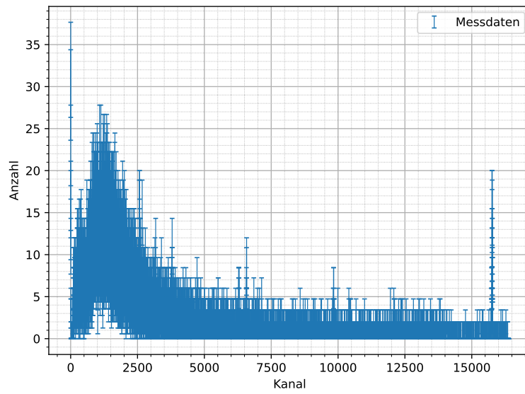
Abbildung 6.7: Mit HPGe-Detektor aufgenommenes Untergrundspektrum ohne Probe mit Fehler der Messanzahl N von \Delta N = \sqrt{N} , welches von den Messungen mit Probe in der weiteren Auswertung immer abgezogen wird. Messdauer: t = 300 s. Aufgrund der gleichen Messzeit muss jeweils keine Normierung der Daten erfolgen.
