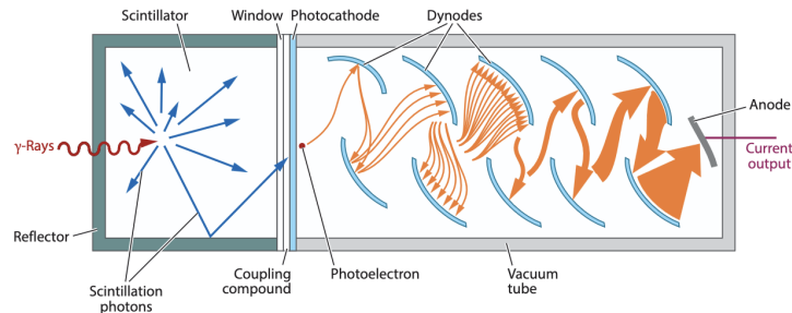
Abbildung 1.1: Aufbau des Szintillationsdetektors mit angeschlossener PMT. Abbildung entnommen aus [8, S. 250].
