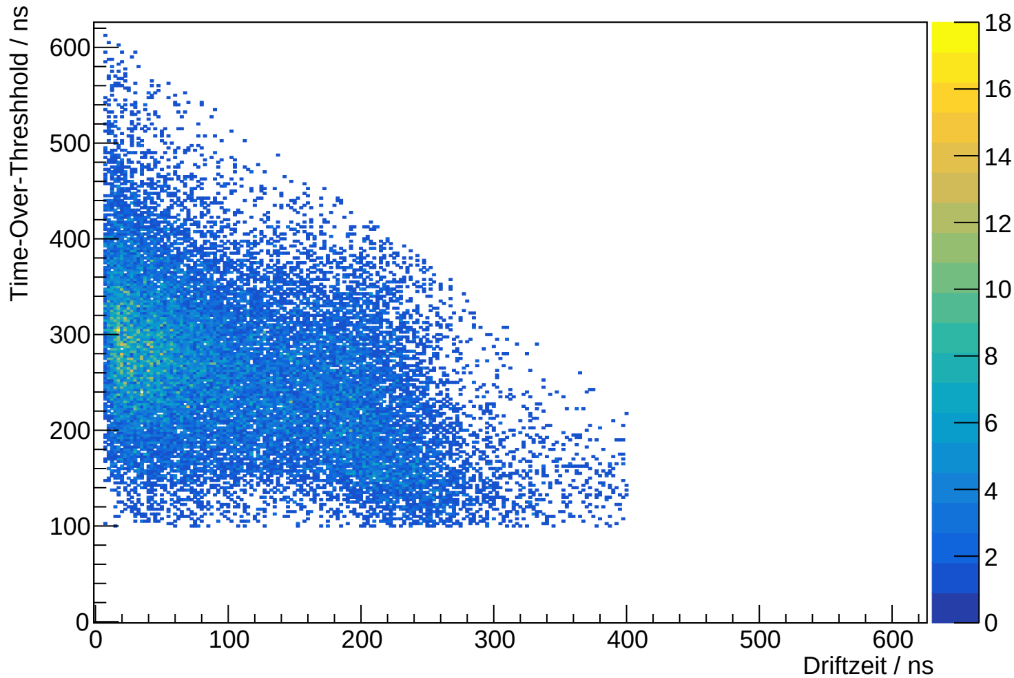
Driftzeit / TOT Relation
