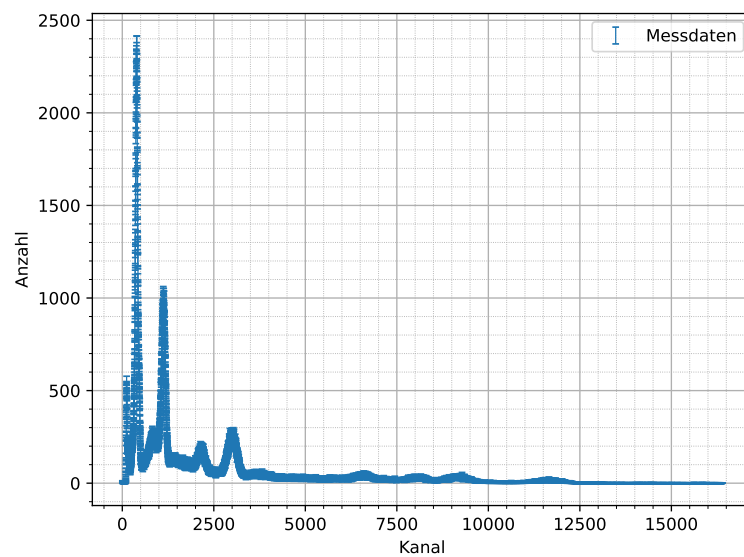
Abbildung 8.6: Mit NaI-Detektor aufgenommenes Spektrum von ^{152}\text{Eu} mit Fehler der Messanzahl N von \Delta N = \sqrt{N} , Messdauer: t = (400,0 \pm 0,5) s.
