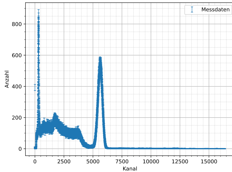
Abbildung 8.5: Mit NaI-Detektor aufgenommenes Spektrum von ^{137}\text{Cs} mit Fehler der Messanzahl N von \Delta N = \sqrt{N} , Messdauer: t = (400,0 \pm 0,5) s.
