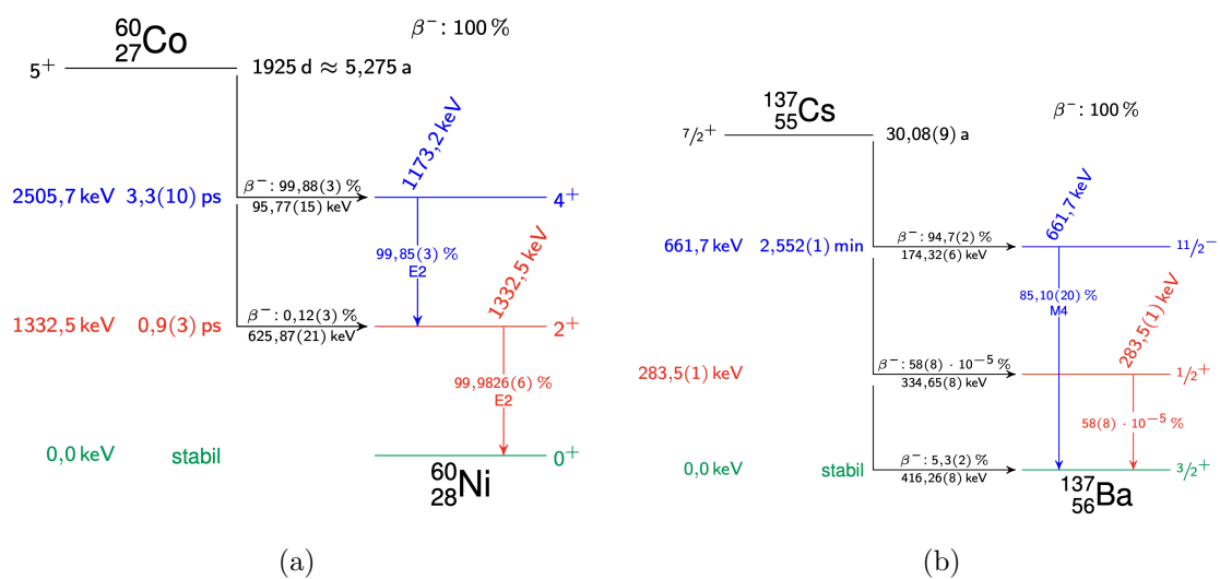
Abbildung 8.13: a) Zerfallsschema von ^{60}\text{Co} , entnommen aus[15, S. 8]. und b) Zerfallsschema von ^{137}\text{Cs} , entnommen aus[15, S. 8].
