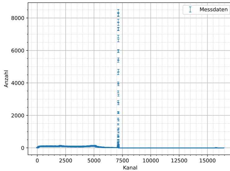
Abbildung 8.9: Mit HPGe-Detektor aufgenommenes Spektrum von ^{137}\text{Cs} mit Fehler der Messanzahl N von \Delta N = \sqrt{N} , Messdauer: t = (300,0 \pm 0,5) \text{ s} .
