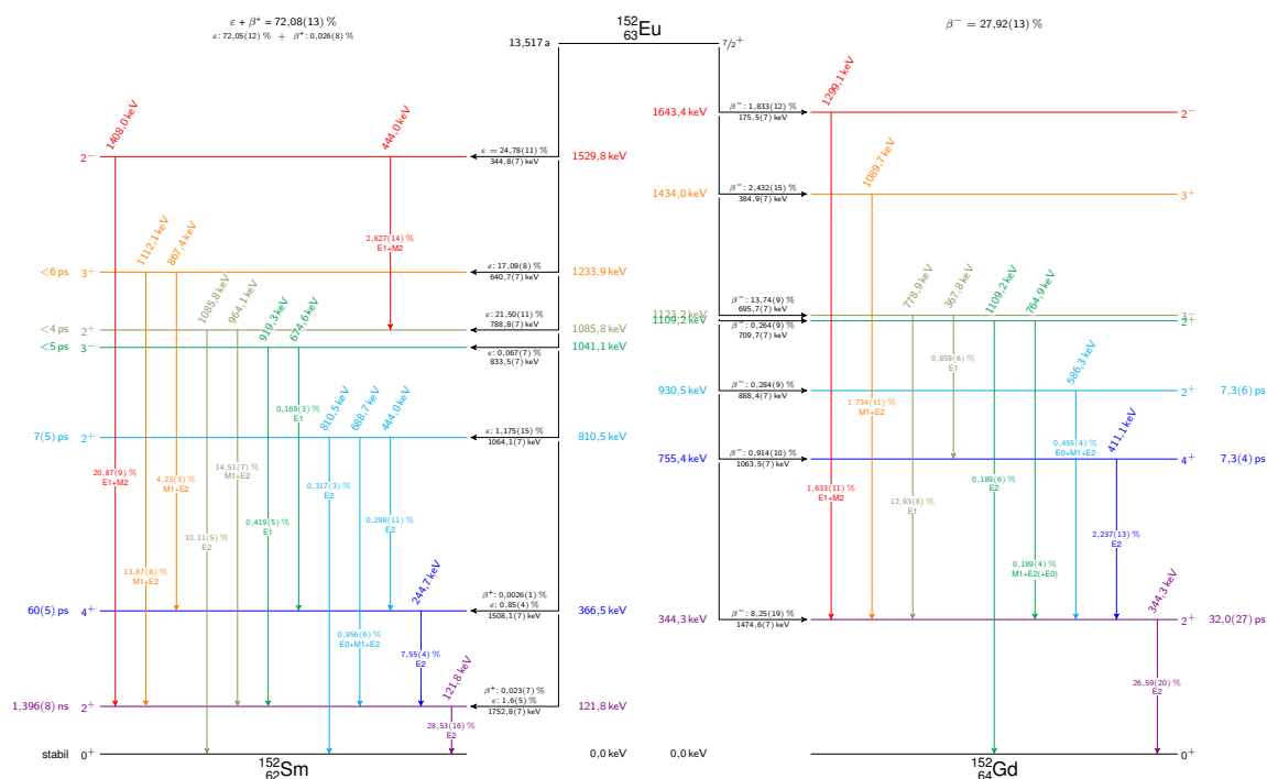
Abbildung 8.14: Zerfallsschema von ^{152}\text{Eu} , entnommen aus[15, S. 9].
