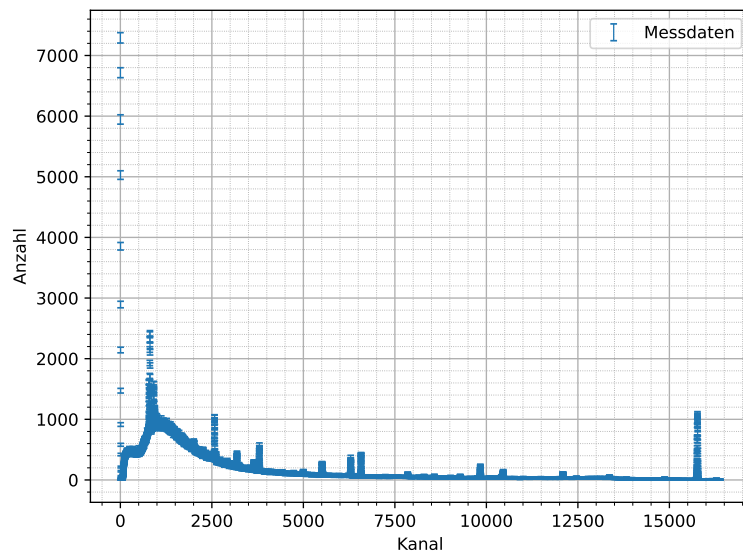
Abbildung 6.12: Mit HPGE-Detektor aufgenommenes Untergrundpektrum für die Bodenprobe, mit Fehler der Messanzahl N von \Delta N = \sqrt{N} , Messdauer: t = 18 h.
