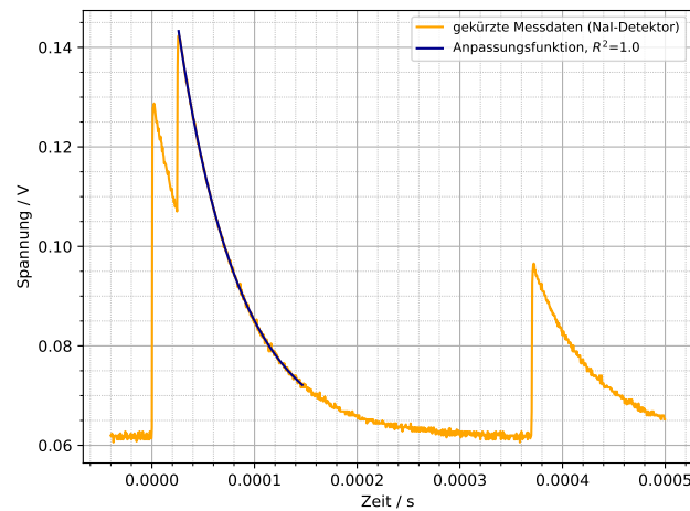
Abbildung 4.1: Ausschnitt der Aufnahme eines Oszilloskopsignals des NaI-Detektors für ^{137}\text{Cs} mit angepasster Exponentialfunktion mit Parametern A = (0,0 \pm 7,8) \cdot 10^3 \text{ V} , b = (-16\,729 \pm 88) \text{ s}^{-1} , c = (0,061\,22 \pm 0,000\,18) \text{ V} , t_0 = (0,0 \pm 1,6) \text{ s} sowie Bestimmtheitsmaß R^2 = 1,000 (letzteres gerundet bis auf die 3. Nachkommastelle).
