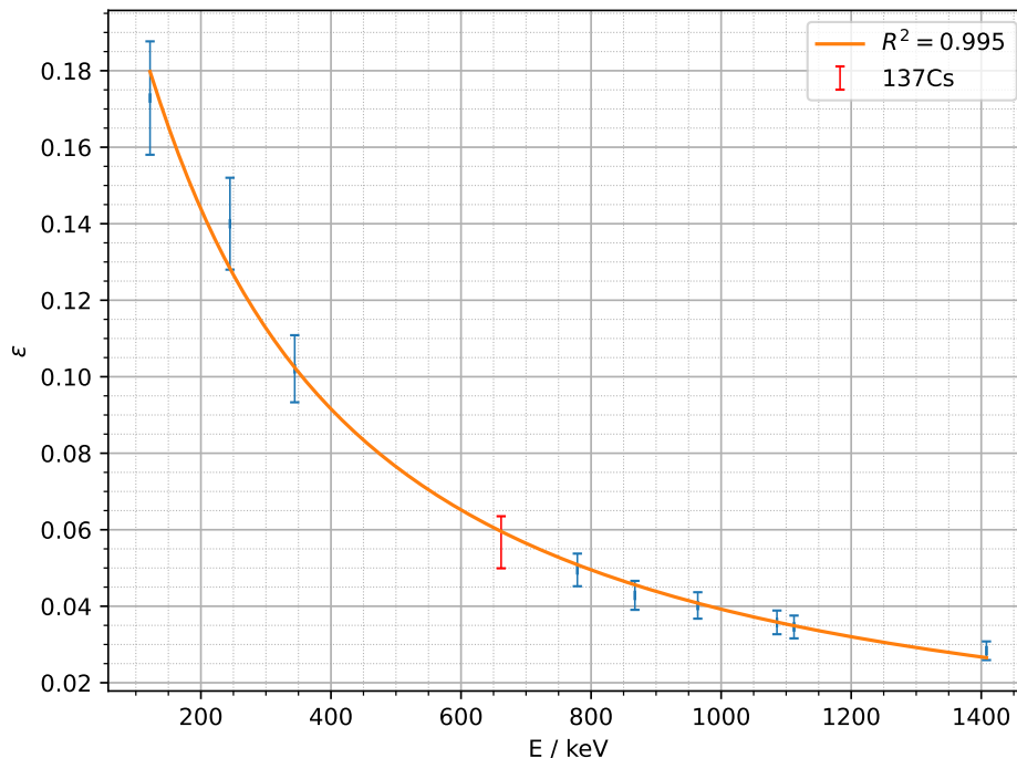
Abbildung 5.1: Effizienzkurve des HPGE Detektors mit Effizienz für Cäsium eingezeichnet
