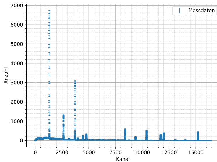
Abbildung 8.10: Mit HPGe-Detektor aufgenommenes Spektrum von ^{152}\text{Eu} mit Fehler der Messanzahl N von \Delta N = \sqrt{N} , Messdauer: t = (300,0 \pm 0,5) s.
