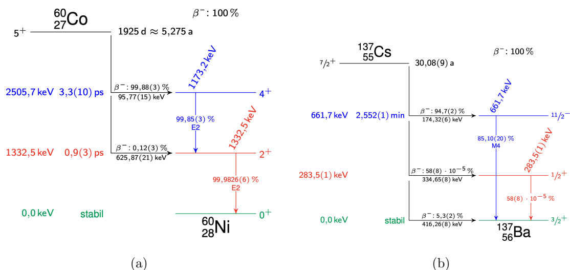
Abbildung 8.13: a) Zerfallsschema von ^{60}\text{Co} , entnommen aus[13, S. 8]. und b) Zerfallsschema von ^{137}\text{Cs} , entnommen aus[13, S. 8].
