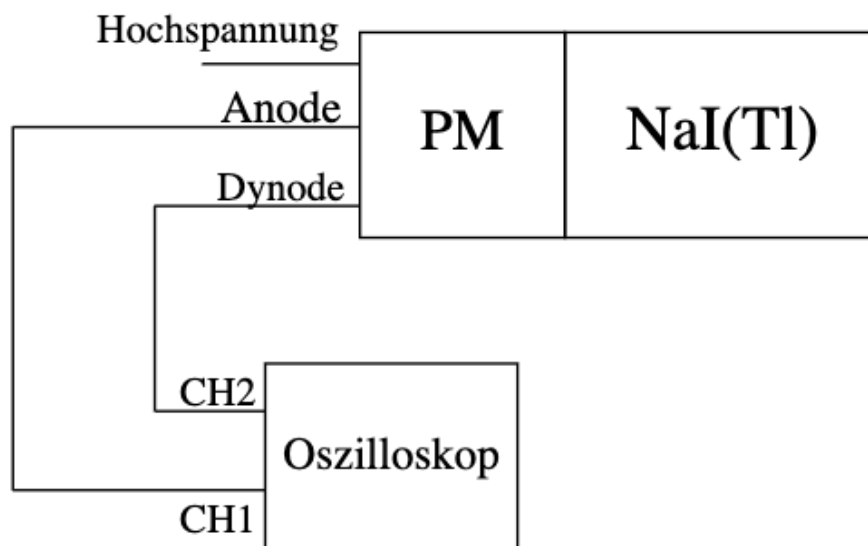
Abbildung 5.1: Schaltplan zur Kontrolle der Fast Pulse
