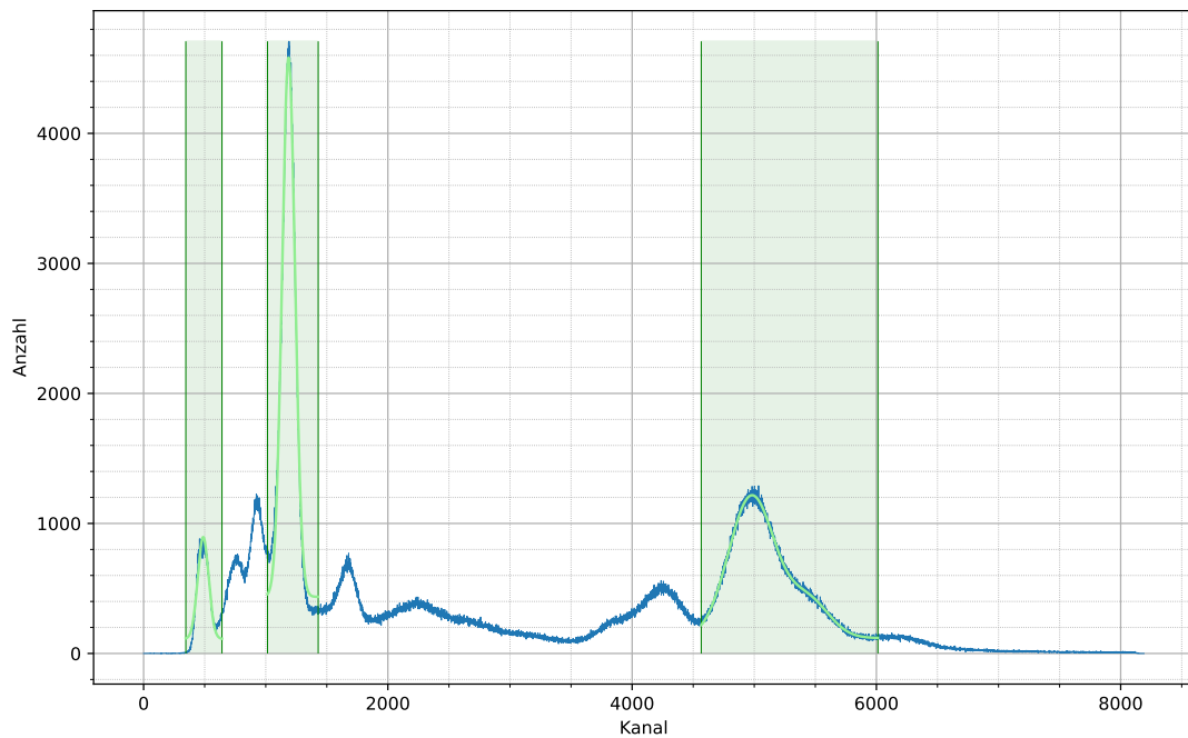
Abbildung 5.8: ^{133}\text{Ba} Spektrum, aufgenommen mit der rechten Seite mit CFD als Gate. Die Parameter der eingezeichneten Anpassungen sind in Tabelle 5.2 gelistet. Die angepassten Linien sind nur zu illustrationszwecken vlrd. die K_{\alpha} , 81,0 keV, 356,0 keV und die 383,8 keV Line. Dies kann anhand durch Vergleich mit Tabelle 4.6 gesehen werden.
