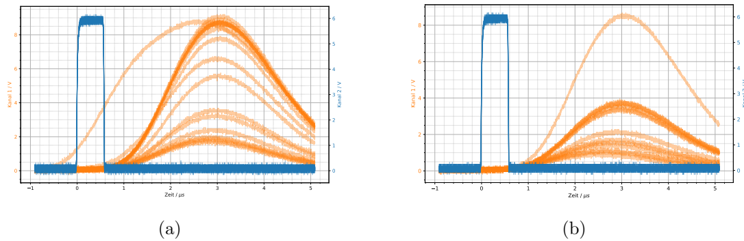
Abbildung 3.8: a) Oszillogramme einiger Pulse mit dem initial eingestellten coarse Gain von 50 für den linken Detektor. Man erkennt eine häufung von Signalen mit einer Amplitude von ca. 8,5 V und b) mit coarse Gain von 20 ist die Anhäufung auf knapp unter ca. 4 V gefallen.
