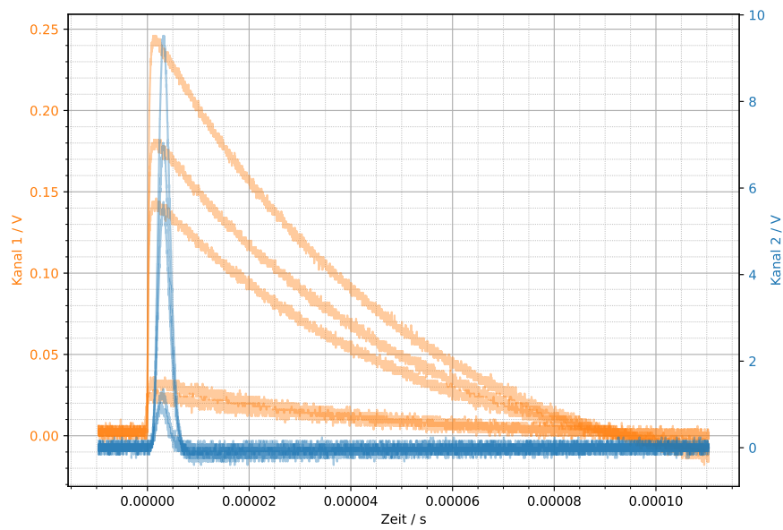
Abbildung 2.2: Slow-Pulse vom Linken Szintillator, auf Kanal 1 direkt am Szintillator abgegriffen, Kanal 2 Hinter dem Hauptverstärker.
