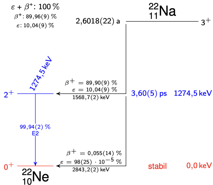
Abbildung 8.3: Zerfallsschemata für ^{22}\text{Na} in ^{22}\text{Ne} . Abbildung entnommen aus [20, S. 9], basierend auf Daten von [15]
