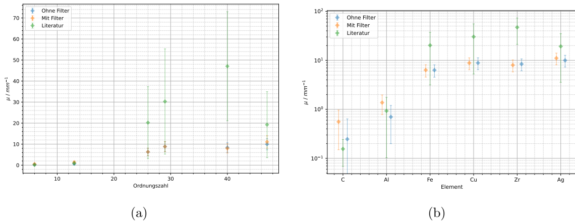
Abbildung 5.2: a) Berechnete Abschkirmungskoeffizienten mit Referenzwerten nach Ordnungszahl 5.3 und b) mit Logarithmierter Y-Achse und Auftragung pro Element.
