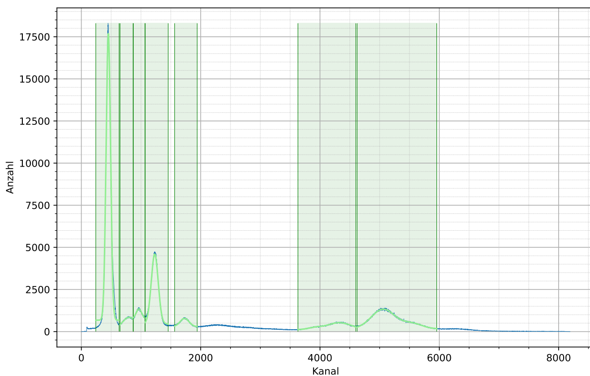
Abbildung 3.6: Mit der rechten Seite Aufgenommenes ^{133}\text{Ba} Spektrum mit angepassten Gaußkurven
