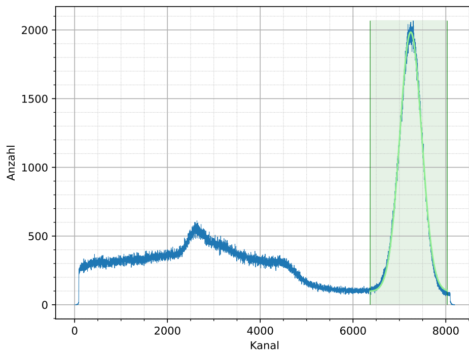
Abbildung 3.5: Mit der rechten Seite Aufgenommenes ^{22}\text{Na} Spektrum mit angepassten Gaußkurven
