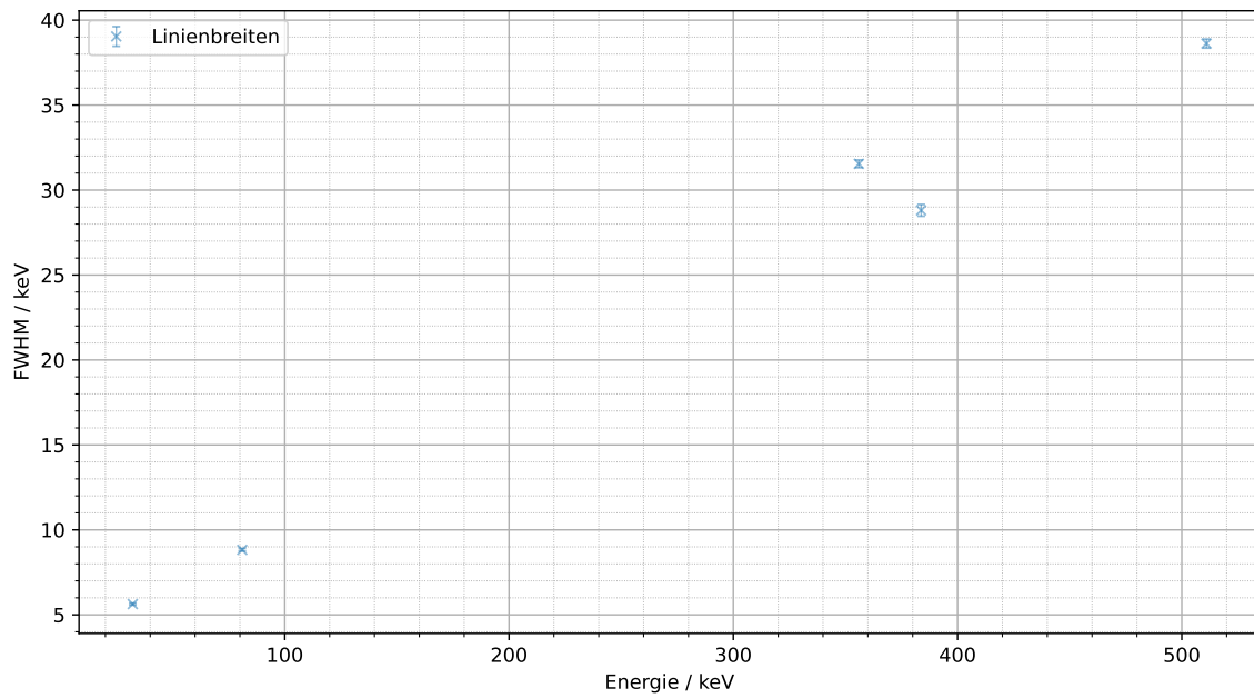
Abbildung 3.4: Linienbreiten gegen Energie der Linien des Linken Szintillators.
