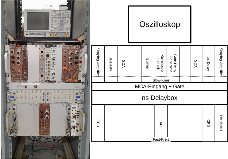
Abbildung 5.1: Anordnung der NIMs in den beiden Reihen, Abbildung entnommen von [5].
