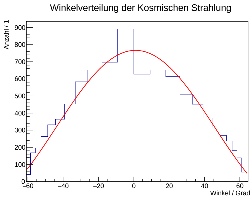
Abbildung 8.2: Winkelverteilung der kosmischen Strahlung, mit Anpassungsfunktion nach Gl (8.3), \chi^2_{\text{red}} = 4.2
