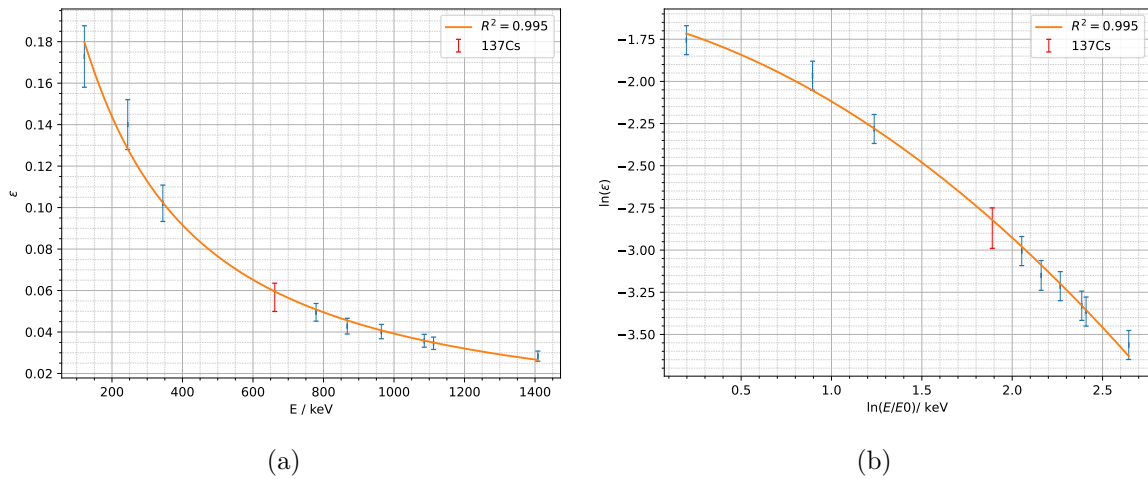
Abbildung 5.1: a) Effizienzkurve des HPGE Detektors mit Effizienz für Cäsium und Anpassungsfunktion eingezeichnet und b) Auftragung der Daten nach (5.8) an denen die Anpassung durchgeführt wurde.
