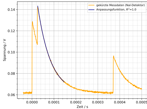
Abbildung 7.1: Ausschnitt der Aufnahme eines Oszilloskopsignals des NaI-Detektors für ^{137}\text{Cs} mit angepasster Exponentialfunktion mit Parametern A = (0,0 \pm 7,8) \cdot 10^3 \text{ V} , b = (-16\,729 \pm 88) \text{ s}^{-1} , c = (0,061\,22 \pm 0,000\,18) \text{ V} , t_0 = (0,0 \pm 1,6) \text{ s} sowie Bestimmtheitsmaß R^2 = 1,000 (letzteres gerundet bis auf die 3. Nachkommastelle).
