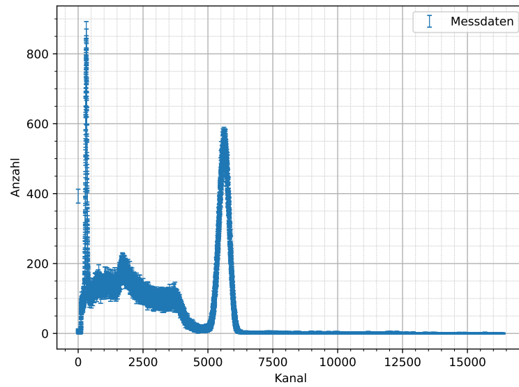
Abbildung 7.5: Mit NaI-Detektor aufgenommenes Spektrum von ^{137}\text{Cs} mit Fehler der Messanzahl N von \Delta N = \sqrt{N} , Messdauer: t = 400 s.
