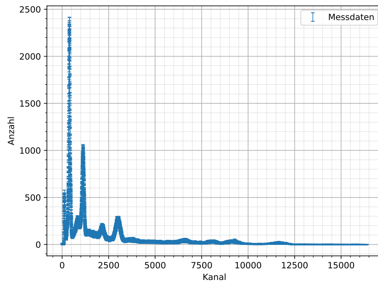
Abbildung 7.6: Mit NaI-Detektor aufgenommenes Spektrum von ^{152}\text{Eu} mit Fehler der Messanzahl N von \Delta N = \sqrt{N} , Messdauer: t = 400 s.
