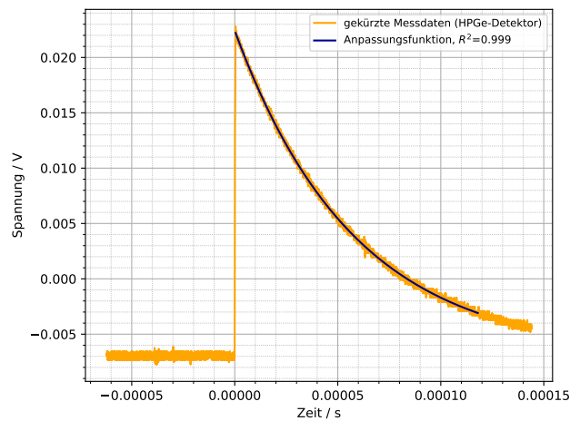
Abbildung 7.2: Ausschnitt der Aufnahme eines Oszilloskopsignals des HPGe-Detektors für ^{137}\text{Cs} mit angepasster Exponentialfunktion mit Parametern A = (0,0 \pm 1,6) \cdot 10^3 \text{ V} , b = (-17\,327 \pm 25) \text{ s}^{-1} , c = (-0,006\,880 \pm 0,000\,018) \text{ V} , t_0 = (0,00 \pm 0,87) \text{ s} sowie Bestimmtheitsmaß R^2 = 0,999 .
