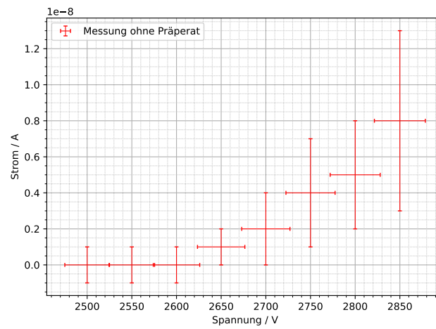
Abbildung 6.3: Darstellung des Stroms durch die Driftkammer I_D ohne Quelle. Man erkennt, dass sich der Strom im Rahmen der Messunsicherheit nur sehr geringfügig mit U_D verändert.
