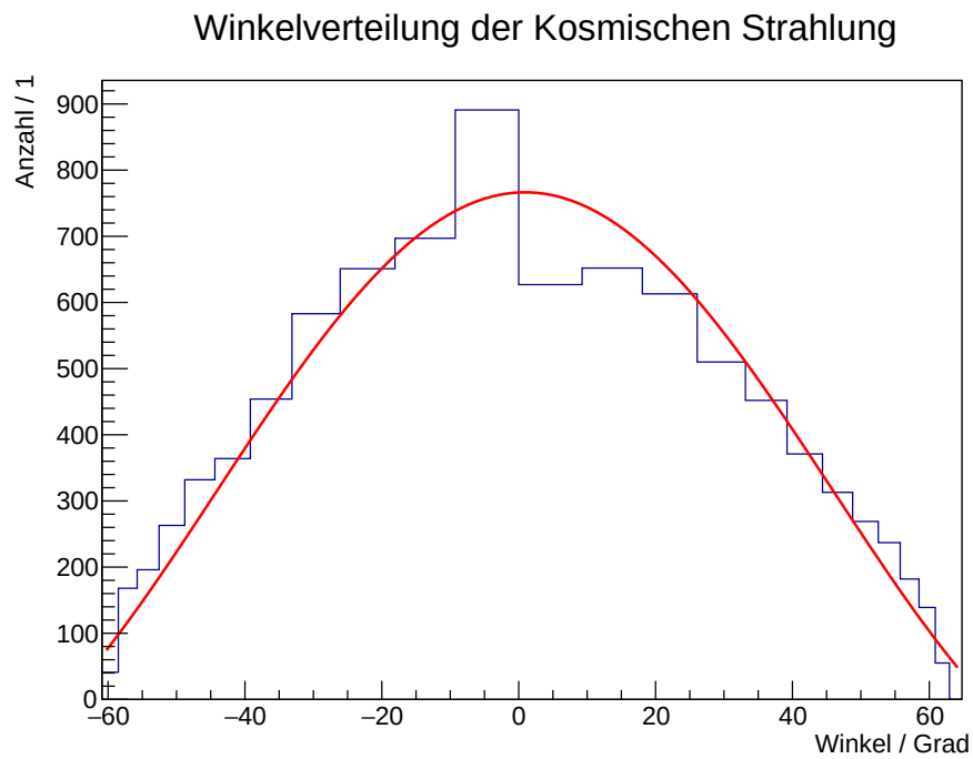
Abbildung 8.2: Winkelverteilung der kosmischen Strahlung, mit Anpassungsfunktion nach Gl (8.3), \chi^2_{red} = 4.2
