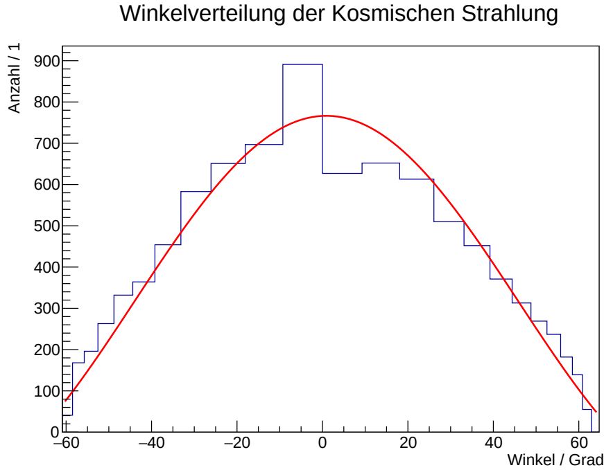
Abbildung 8.2: Winkelverteilung der kosmischen Strahlung, mit Anpassungsfunktion nach Gl (8.3), \chi_{\text{red}}^2 = 4.2
