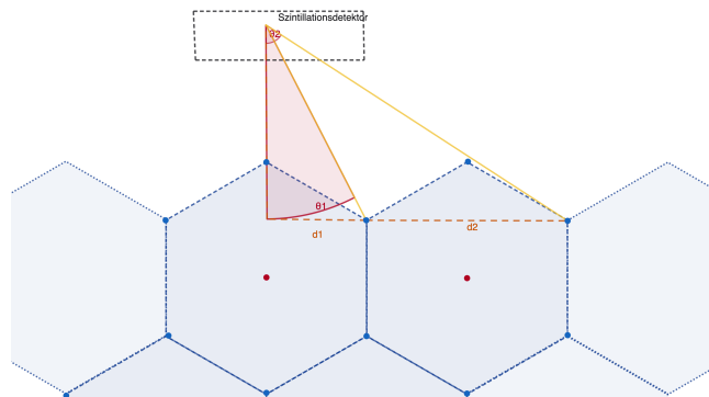
Abbildung 8.1: Skizze der Berechnung der Winkelbereiche zu jeder Zelle
