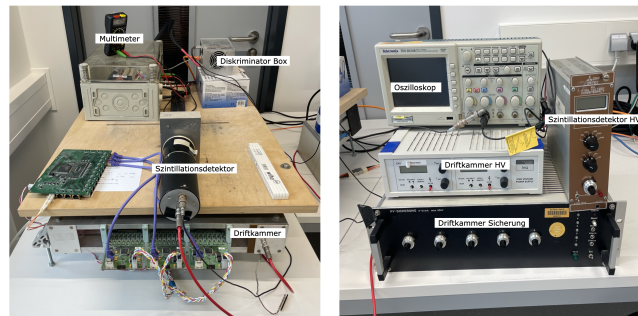
Abbildung 5.4: Messaufbau zur Langzeitmessung. Das Multimeter (DMM) wird für diese Messung nicht benötigt, es wurde nur für die Strommessung genutzt. Abbildung entnommen von [13]
