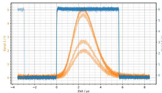
Abbildung 2.11: DA Signal (Ch1) gegen GDG Ausgang (Ch2) für den rechten Detektor, es ist keine Anpassung der GDG Einstellungen nötig.
