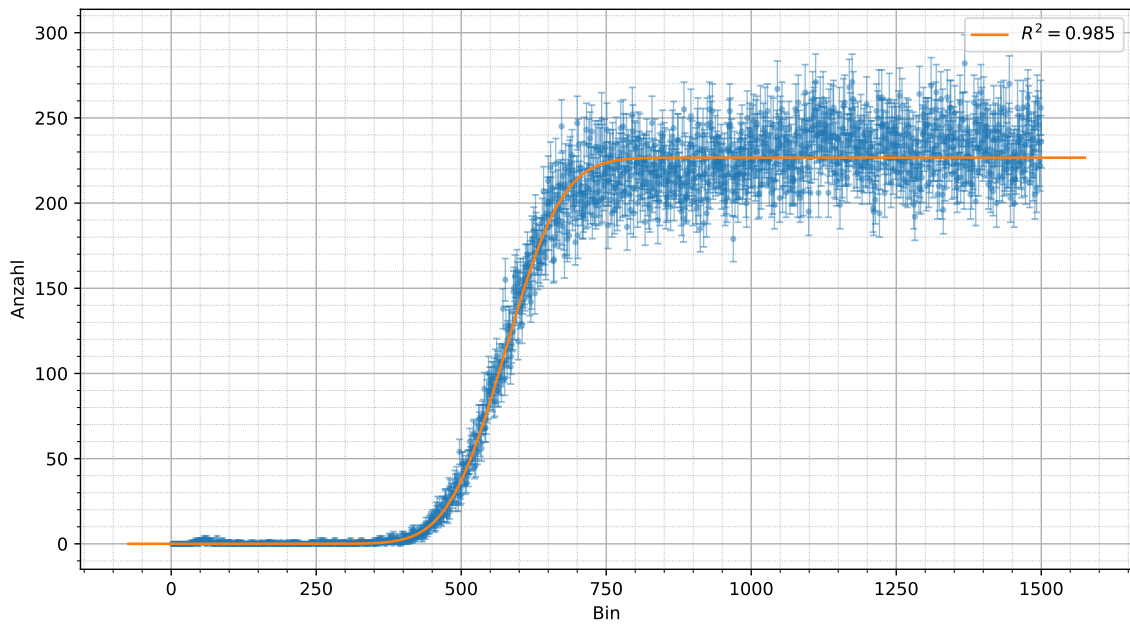
Abbildung 4.5: Anpassung zur Bestimmung der linken CFD Schwelle, an die ersten 1500 Kanäle.
