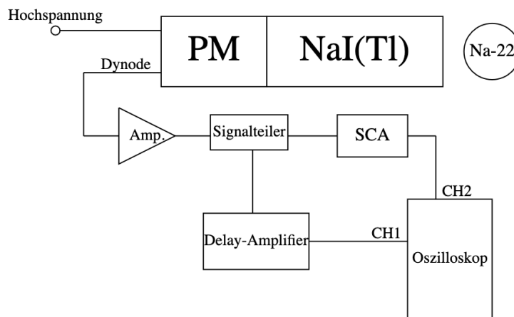
Abbildung 2.6: Schaltplan zur Einstellung der Verstärkung des Hauptverstärkers.
