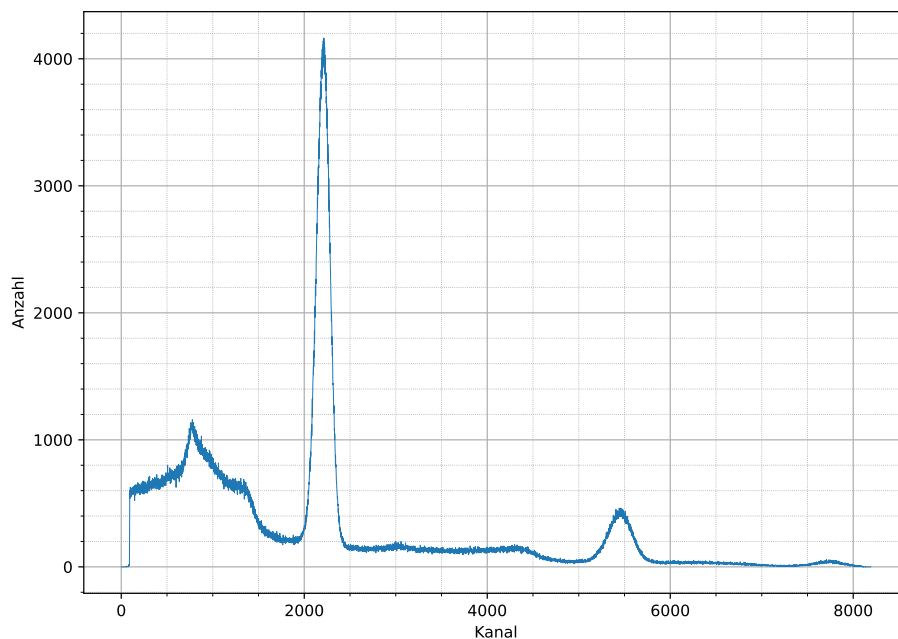
Abbildung 2.14: Energiespektrum der ^{22}\text{Na} Quelle am rechten Slow-Kreis. Zur besseren Lesbarkeit wurde auf Fehlerbalken verzichtet.
