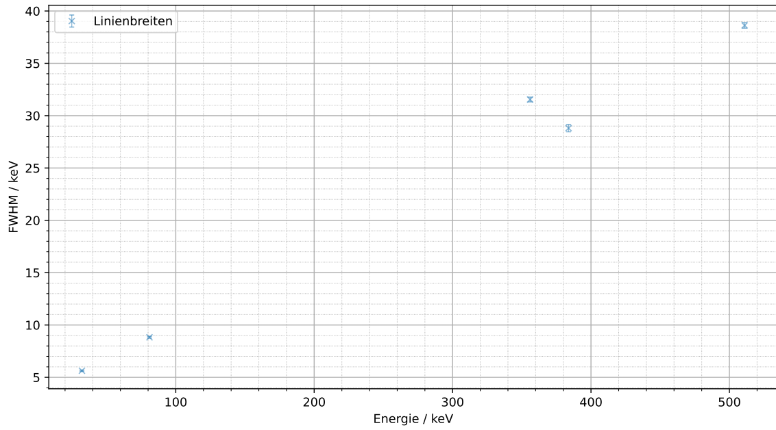
Abbildung 3.7: Linienbreiten gegen Energie der Linien des Linken Szintillators.
