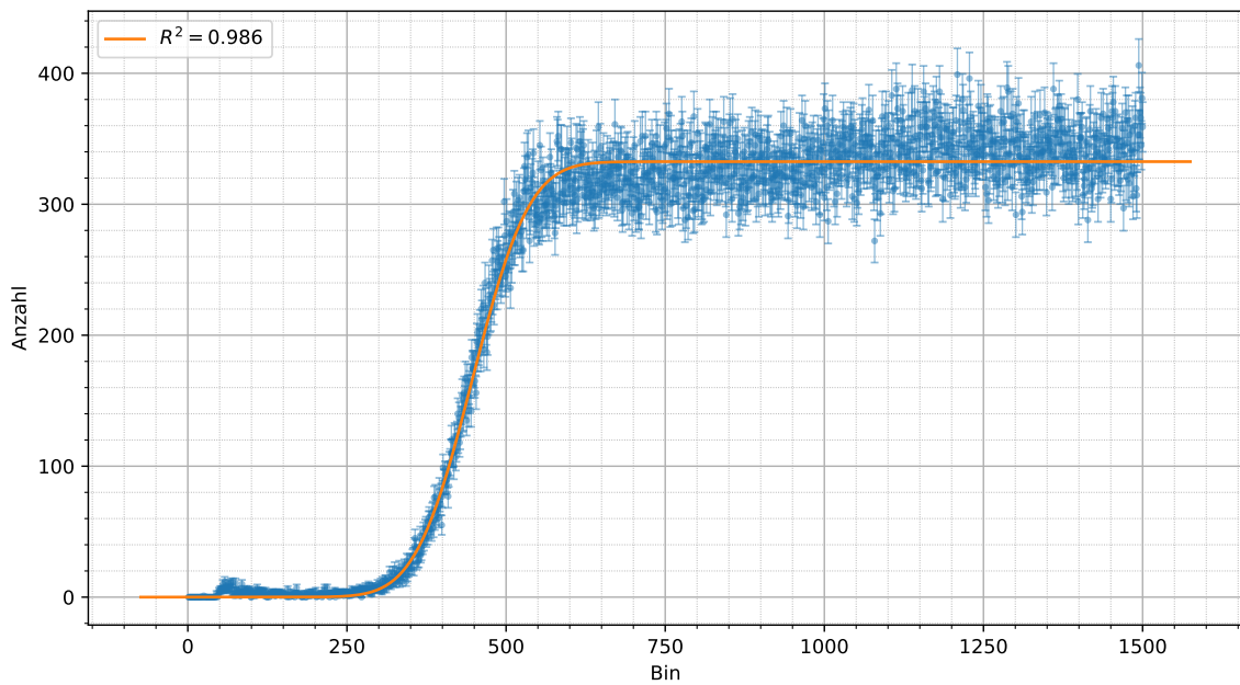
Abbildung 4.6: Anpassung zur Bestimmung der linken CFD Schwelle, an die ersten 1500 Kanäle.
