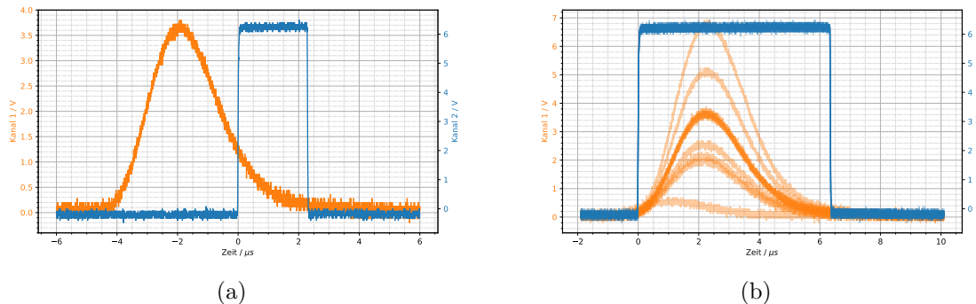
Abbildung 2.9: a) DA Signal (Ch1) gegen GDG Ausgang (Ch2) für den linken Detektor, vor Anpassung der GDG Einstellungen und b) nach Anpassung der GDG Einstellungen.
