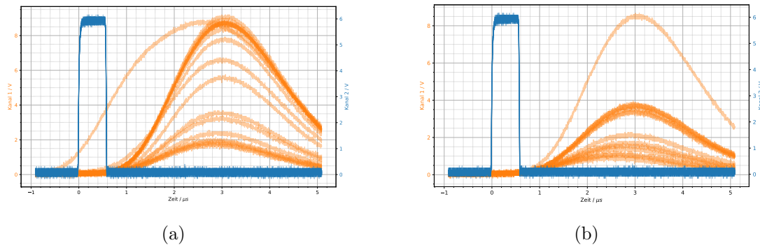
Abbildung 2.8: a) Oszillogramme einiger Pulse mit dem initial eingestellten coarse Gain von 50 für den linken Detektor. Man erkennt eine häufung von Signalen mit einer Amplitude von ca. 8,5 V und b) mit coarse Gain von 20 ist die Anhäufung auf knapp unter ca. 4 V gefallen.
