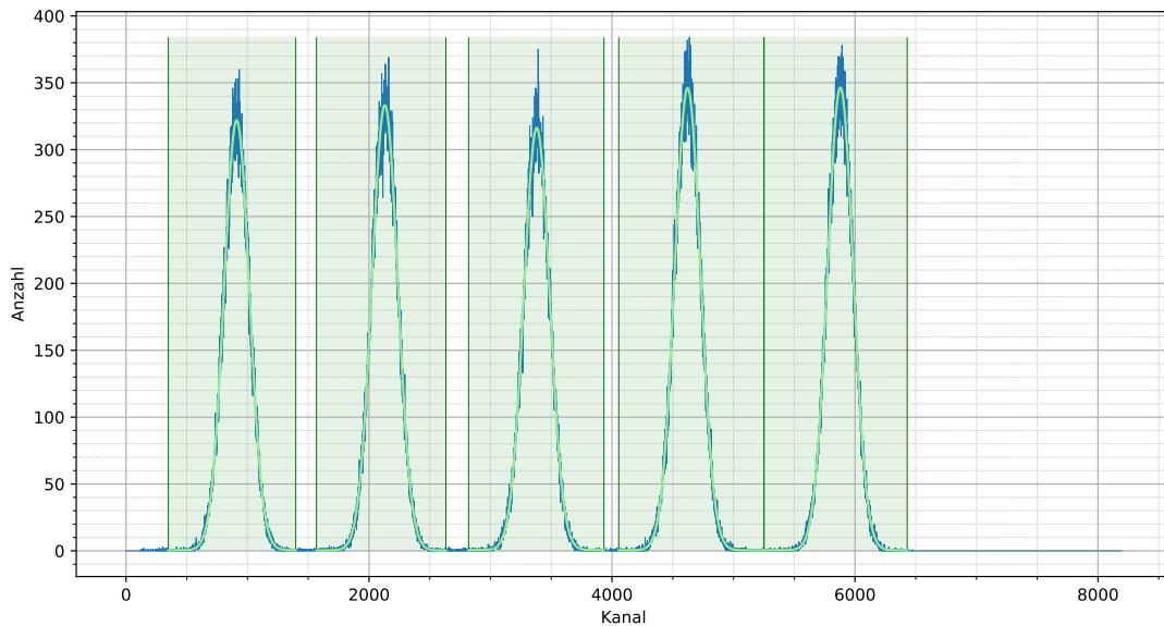
Abbildung 6.1: Promptkurve mit angepassten Gaußfunktionen.
