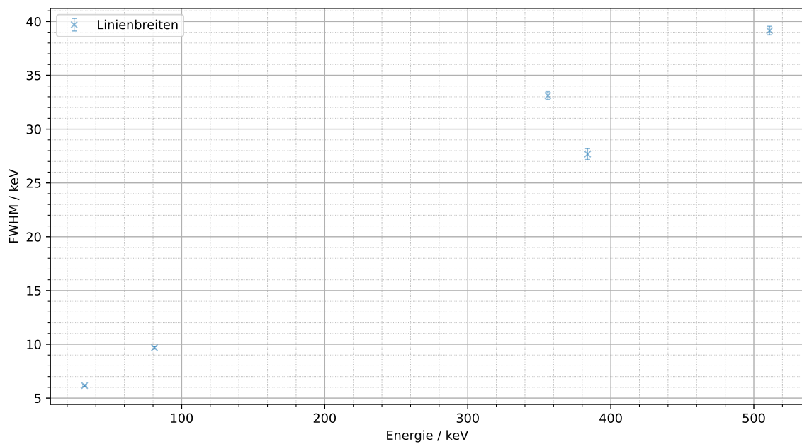
Abbildung 3.8: Linienbreiten gegen Energie der Linien des rechten Szintillators.
