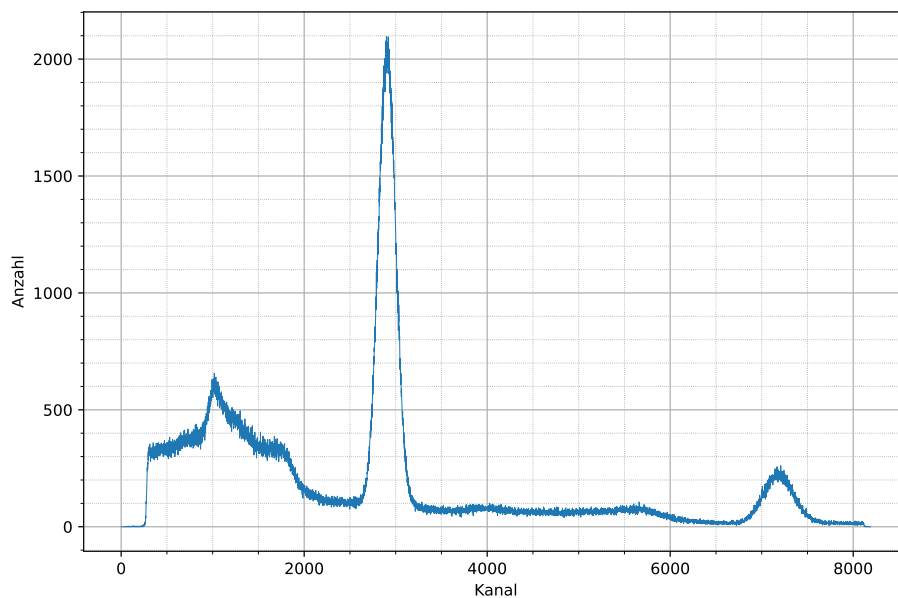
Abbildung 2.13: Energiespektrum der ^{22}\text{Na} Quelle am linken Slow-Kreis. Zur besseren Lesbarkeit wurde auf Fehlerbalken verzichtet.
