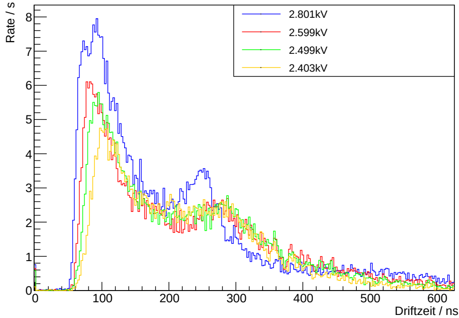
Abbildung 5.1: Driftzeitspektren mit verschiedenen Einstellungen der Hochspannung der Driftkammer U_D , bei \text{CSR\_THR}=0x0020 , \text{CSR\_DDC}=0x0023 .
