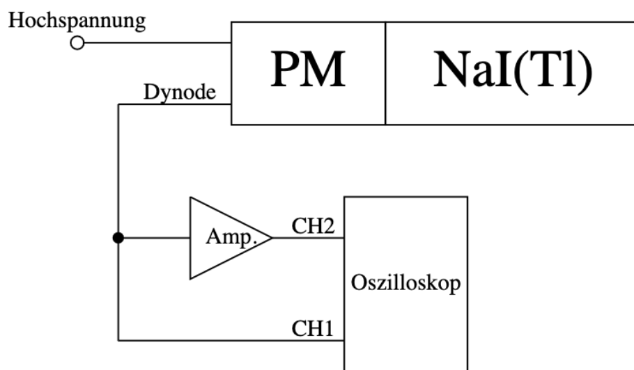
Abbildung 2.1: Aufbau zur Kontrolle der Pulse im Slow-Kreis
