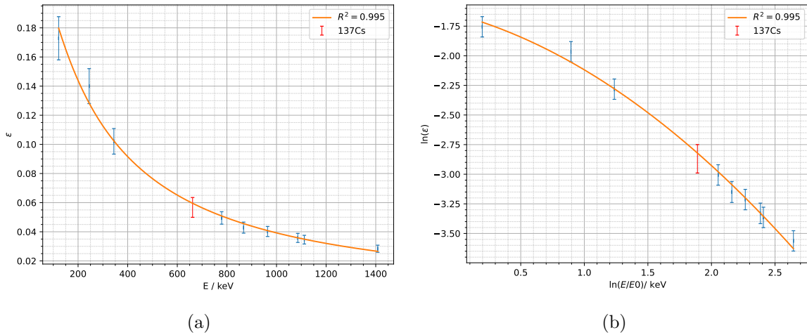
Abbildung 7.1: a) Effizienzkurve des HPGE Detektors mit Effizienz für Cäsium und Anpassungsfunktion eingezeichnet und b) Auftragung der Daten nach (7.8) an denen die Anpassung durchgeführt wurde.
