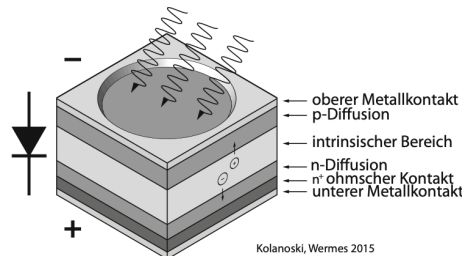
Abbildung 2.3: Schematischer Aufbau einer PiN-Diode mit p- und n-dotierten Bereichen sowie intrinsischer Zone und Schaltungsrichtung. Abbildung entnommen aus [4, S. 422].
