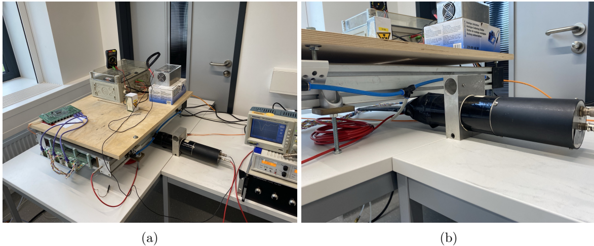
Abbildung 3.1: a) Aufnahme des Aufbaus zur Strommessung mit Szintillator mittig unter dem Schlitz in der Driftkammer zusammen mit (hier neben dem Schlitz platzierter) ^{90}\text{Sr} -Quelle auf der Driftkammer. Die Elektronen, die von ^{90}\text{Sr} emittiert werden, können das Holz neben dem Schlitz nicht passieren, dies entspricht also dem Messfall ohne Quelle. und b) Nahaufnahme des Szintillators unterhalb des Schlitzes, was für Abschnitt [ref abschnitt kalibration rate] wichtig ist.
