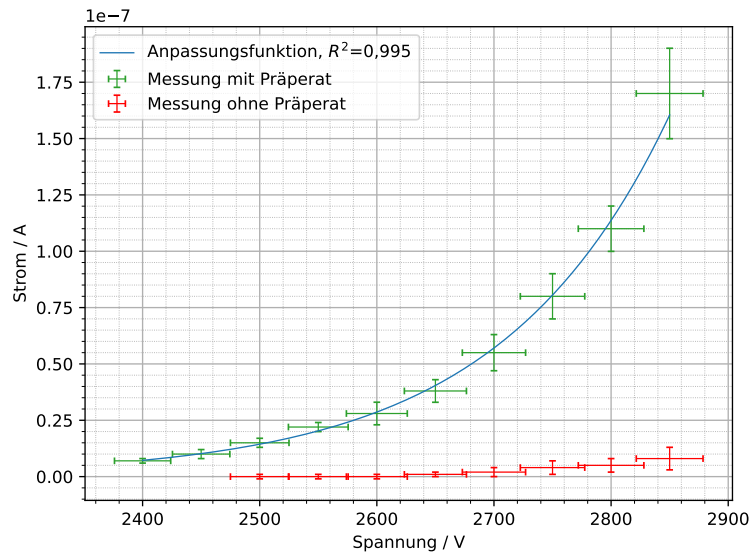
Abbildung 3.2: Darstellung des Verlaufs des Stroms durch die Driftkammer I_D (gemessen am äußersten Pin der unteren Lage) abhängig von der Versorgungshochspannung U_D der Driftkammer mit (in grün) und ohne (in rot) ^{90}\text{Sr} -Quelle. Es ist eine Exponentialfunktion der Form I_D = C \exp\{aU_D\} an die Messwerte mit Quelle angepasst (in blau), das Bestimmtheitsmaß R^2 = 0,995 zeigt eine sehr gute Anpassungsgüte.
