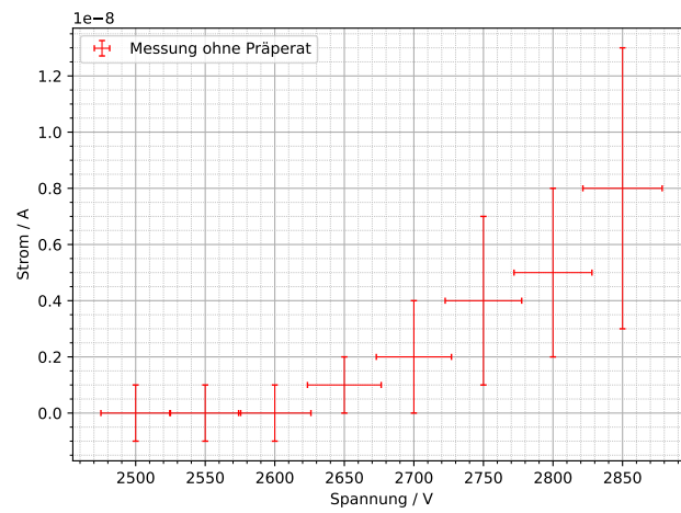
Abbildung 4.3: Darstellung des Stroms durch die Driftkammer I_D ohne Quelle. Man erkennt, dass sich der Strom im Rahmen der Messunsicherheit nur sehr geringfügig mit U_D verändert.
